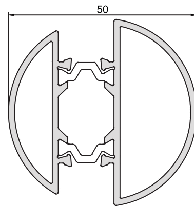
KOD-CODE AT-5566-16
