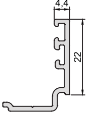
KOD-CODE CC-1044-15 TEORİK AĞIRLIK THEORETICAL WEIGHT 0,212 Kg/m
