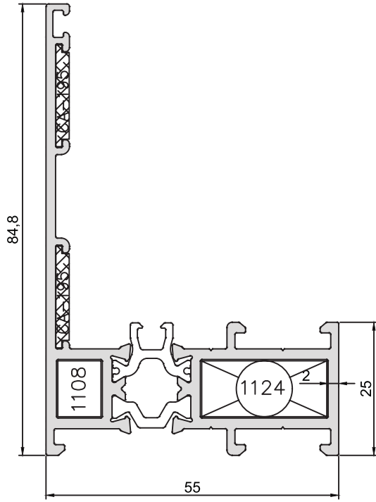
KOD-CODE AT-5515-20 TEORİK AĞIRLIK THEORETICAL WEIGHT 1,407 Kg/m
