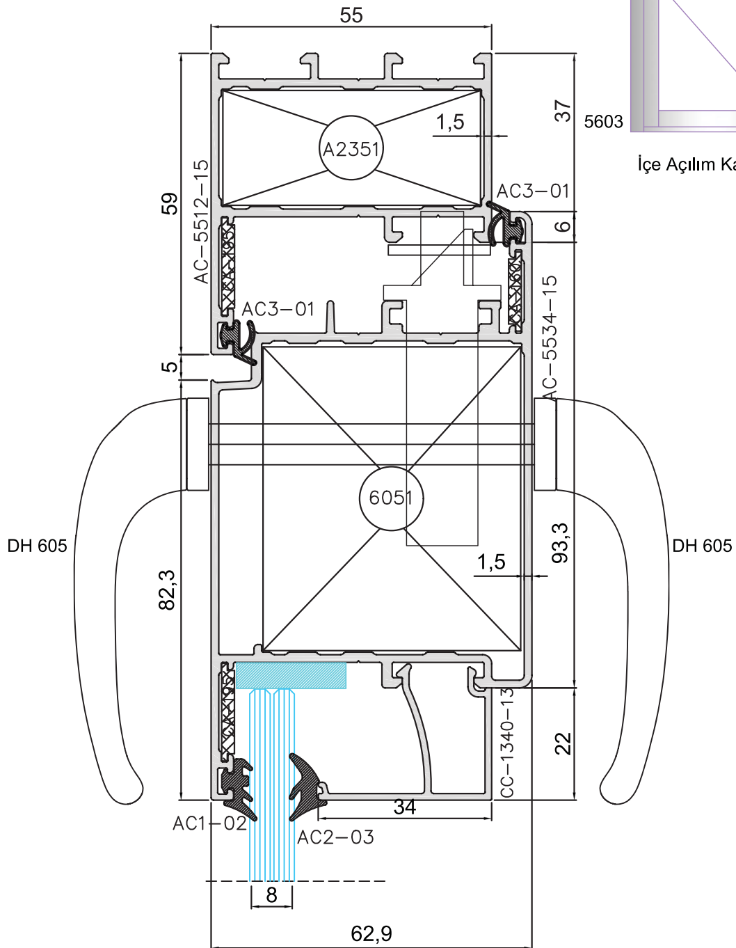
1 Kapı Kilit Detay
