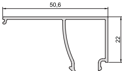
KOD-CODE CC-1506-13 TEORİK AĞIRLIK THEORETICAL WEIGHT 0,378 Kg/m
