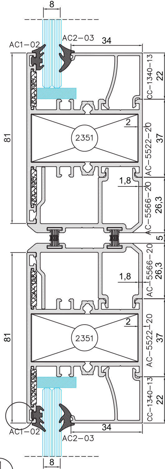
Geniş Çarpma Kapı Kilit Detay
