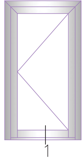
Etek Detayı
