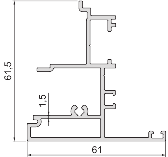
KOD-CODE AC-5562-15 TEORİK AĞIRLIK THEORETICAL WEIGHT 1,061 Kg/m
