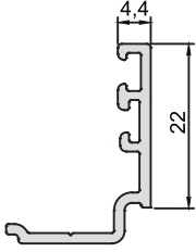
KOD-CODE CC-1044-13 TEORİK AĞIRLIK THEORETICAL WEIGHT 0,212 Kg/m
