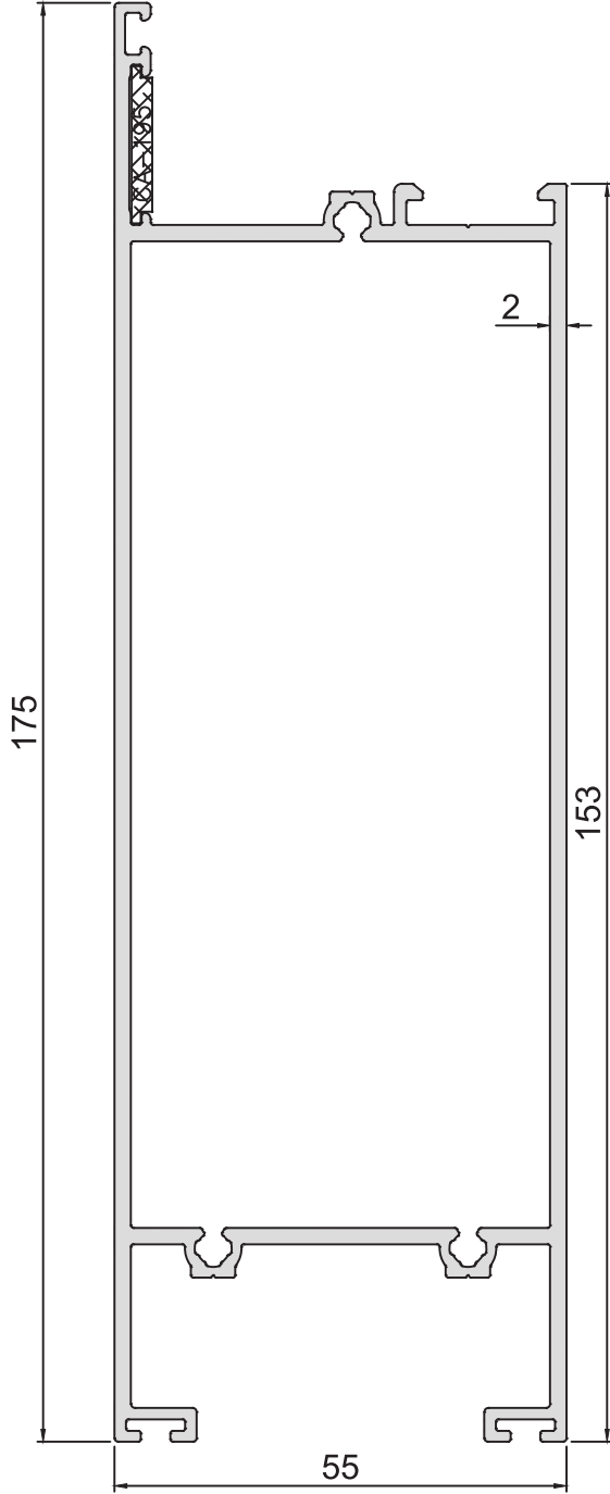
KOD-CODE AC-5554-20 TEORİK AĞIRLIK THEORETICAL WEIGHT 2,548 Kg/m
