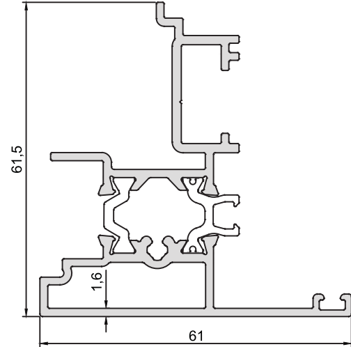
KOD-CODE AT-5562-16
