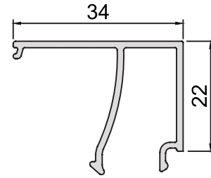
KOD-CODE CC-1340-13 TEORİK AĞIRLIK THEORETICAL WEIGHT 0,320 Kg/m
