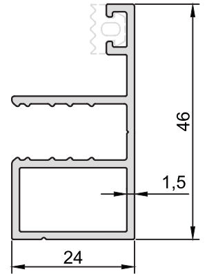
KOD-CODE 8511 TEORİK AĞIRLIK THEORETICAL WEIGHT 0,559 Kg/m
