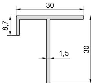
KOD-CODE 1059 TEORİK AĞIRLIK THEORETICAL WEIGHT 0,265 Kg/m
