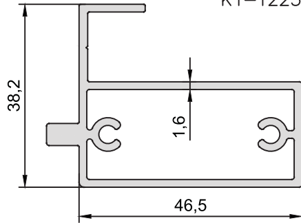
KOD-CODE KT-5023-00 TEORİK AĞIRLIK THEORETICAL WEIGHT 0,914 Kg/m
