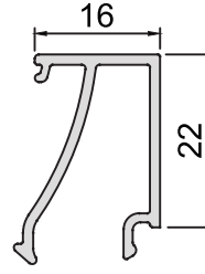
KOD-CODE CC-1160-13 TEORİK AĞIRLIK THEORETICAL WEIGHT 0,260 Kg/m
