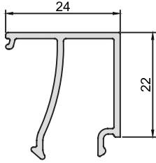
KOD-CODE CC-1240-13 TEORİK AĞIRLIK THEORETICAL WEIGHT 0,285 Kg/m
