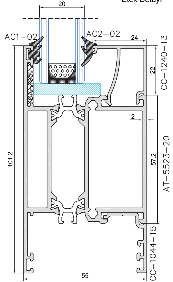
Etek Detayı
