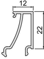
KOD-CODE CC-1120-13 TEORİK AĞIRLIK THEORETICAL WEIGHT 0,254 Kg/m
