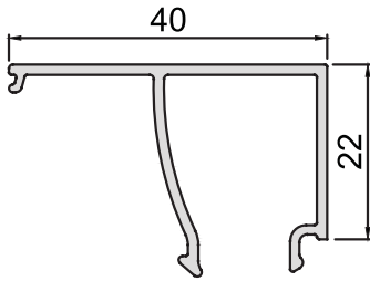
KOD-CODE CC-1400-13 TEORİK AĞIRLIK THEORETICAL WEIGHT 0,341 Kg/m
