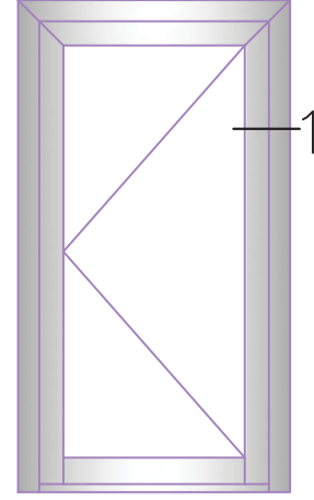
Hemyüz İç Açılır Kapı
