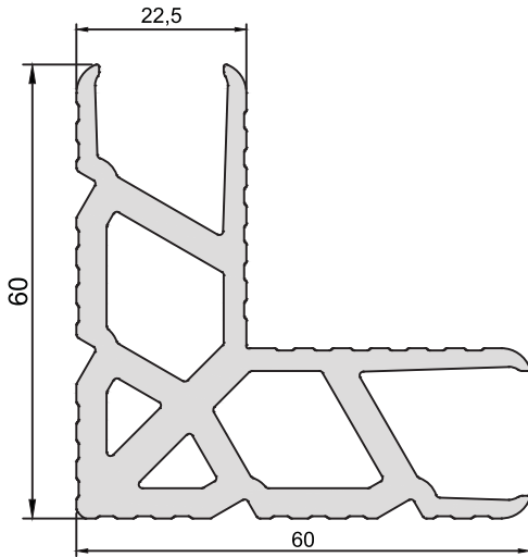
KOD-CODE KT-2225-00 TEORİK AĞIRLIK THEORETICAL WEIGHT 2,543 Kg/m
