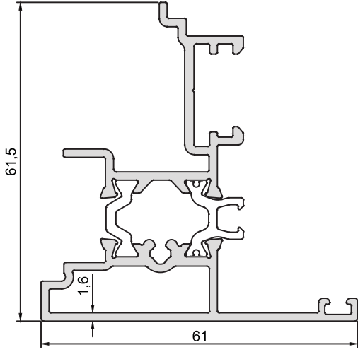
KOD-CODE AT-5561-16
