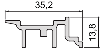
KOD-CODE AC-5575-15 TEORİK AĞIRLIK THEORETICAL WEIGHT 0,332 Kg/m
