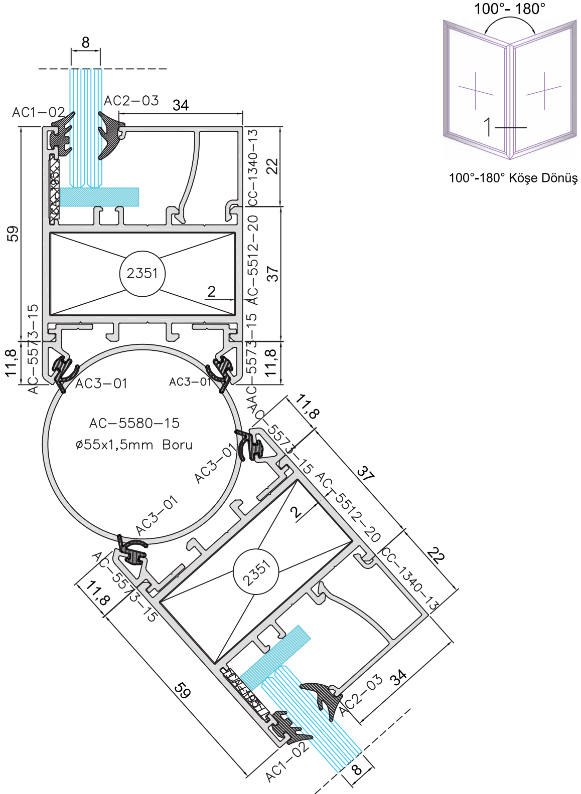
100°-180° Köşe Dönüş Detay
