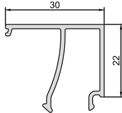
KOD-CODE CC-1300-13 TEORİK AĞIRLIK THEORETICAL WEIGHT 0,305 Kg/m
