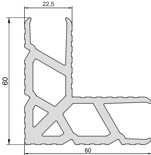
KOD-CODE TEORİK AĞIRLIK KT-2225-00 THEORETICAL WEIGHT 2,543 Kg/m
