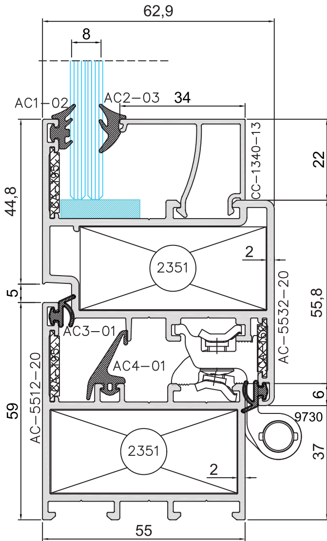
Menteşe Detay
