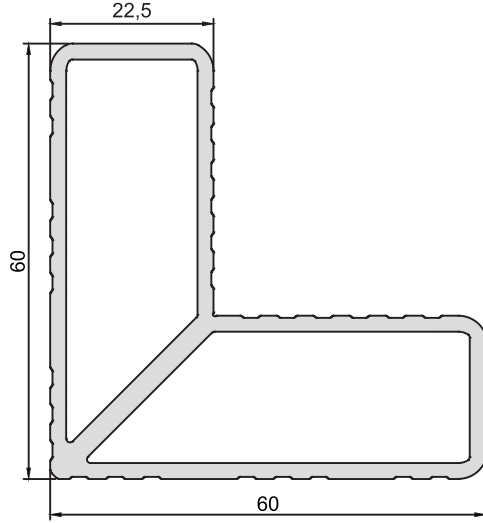
KOD-CODE KT-1225-00 TEORİK AĞIRLIK THEORETICAL WEIGHT 1,508 Kg/m
