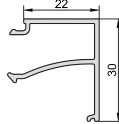
KOD-CODE CC-1300-13 TEORİK AĞIRLIK THEORETICAL WEIGHT 0,305 Kg/m
