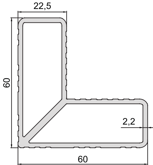
KOD-CODE TEORİK AĞIRLIK KT-1225-00 THEORETICAL WEIGHT 1,508 Kg/m
