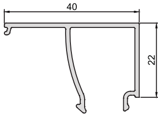
KOD-CODE CC-1400-13 TEORİK AĞIRLIK THEORETICAL WEIGHT 0,341 Kg/m
