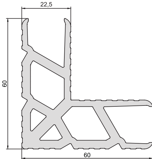
KOD-CODE KT-2225-00 TEORİK AĞIRLIK THEORETICAL WEIGHT 2,543 Kg/m
