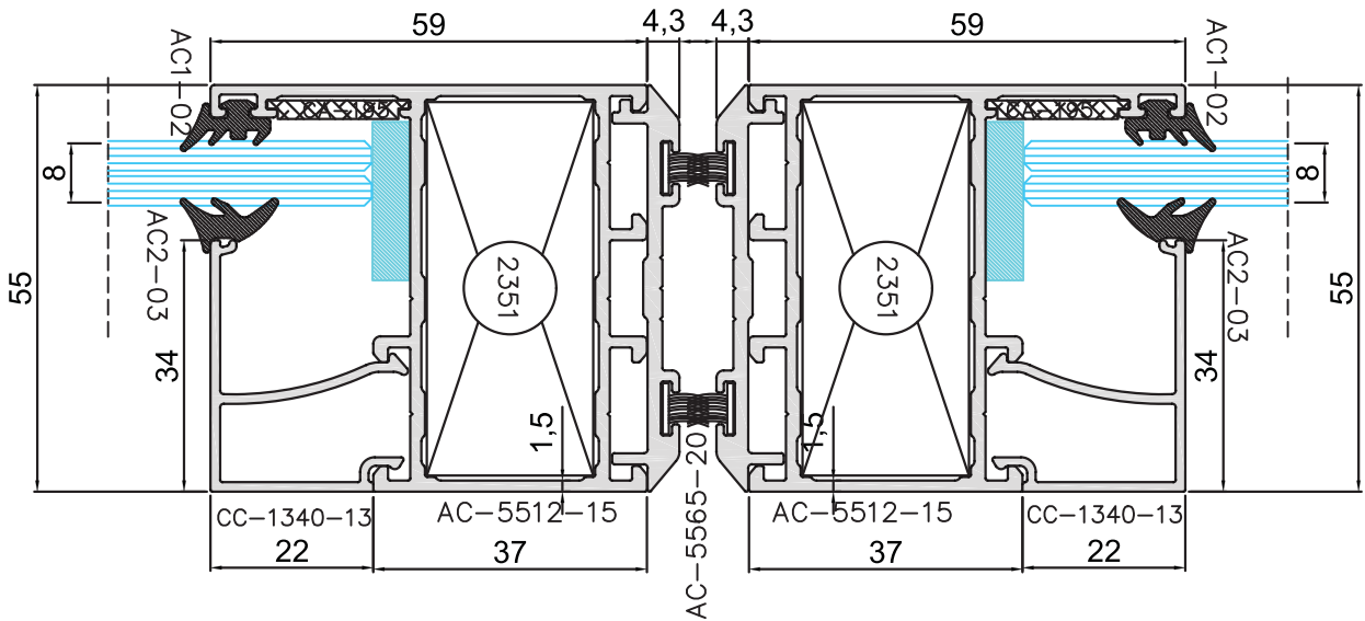
Dar Çarpma Kapı Kilit Detay
