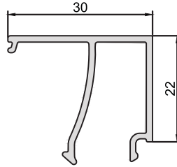
KOD-CODE CC-1300-13 TEORİK AĞIRLIK THEORETICAL WEIGHT 0,305 Kg/m
