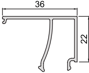
KOD-CODE CC-1360-13 TEORİK AĞIRLIK THEORETICAL WEIGHT 0,327 Kg/m
