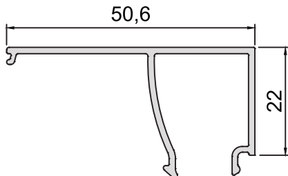
KOD-CODE CC-1506-13 TEORİK AĞIRLIK THEORETICAL WEIGHT 0,378 Kg/m
