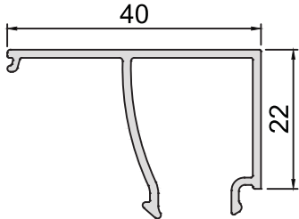
KOD-CODE CC-1400-13 TEORİK AĞIRLIK THEORETICAL WEIGHT 0,341 Kg/m
