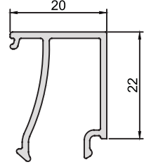
KOD-CODE CC-1200-13 TEORİK AĞIRLIK THEORETICAL WEIGHT 0,270 Kg/m
