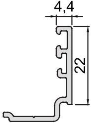
KOD-CODE CC-1044-15 TEORİK AĞIRLIK THEORETICAL WEIGHT 0,212 Kg/m
