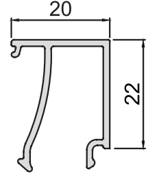
KOD-CODE CC-1200-13 TEORİK AĞIRLIK THEORETICAL WEIGHT 0,270 Kg/m
