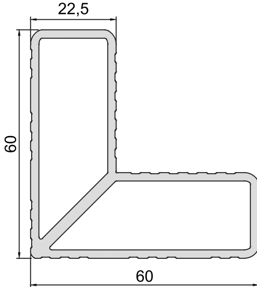
KOD-CODE KT-1225-00 TEORİK AĞIRLIK THEORETICAL WEIGHT 1,508 Kg/m
