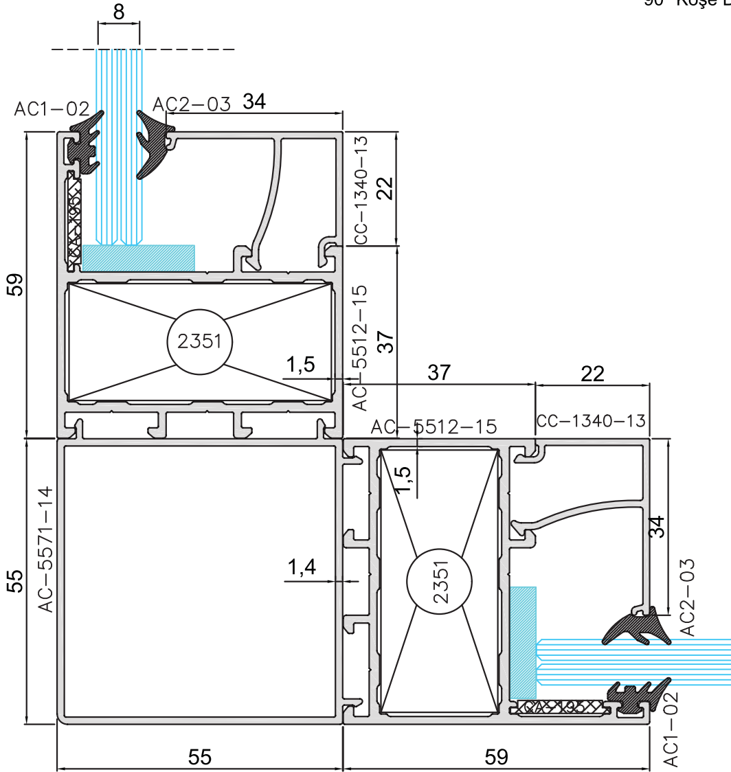
90° Köşe Dönüş
