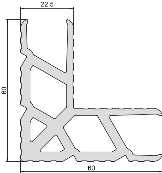
KOD-CODE KT-2225-00 TEORİK AĞIRLIK THEORETICAL WEIGHT 2,543 Kg/m
