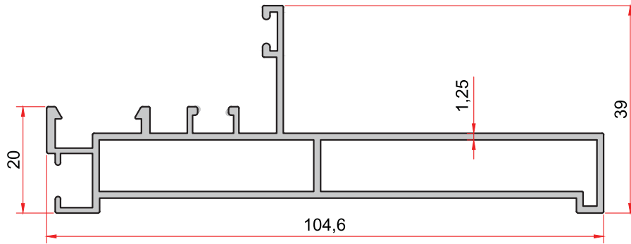
KOD-CODE TEORİK AĞIRLIK THEORETICAL WEIGHT 1076 1,032 Kg/m
