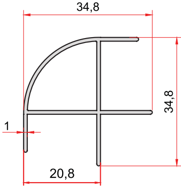
KOD-CODE 1390 TEORİK AĞIRLIK THEORETICAL WEIGHT 0,321 Kg/m
