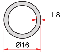
KOD-CODE 1883 TEORİK AĞIRLIK THEORETICAL WEIGHT 0,216 Kg/m
