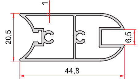
KOD-CODE 1772 TEORİK AĞIRLIK THEORETICAL WEIGHT 0,518 Kg/m
