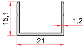
KOD-CODE TEORİK AĞIRLIK THEORETICAL WEIGHT 1481 0,156 Kg/m
