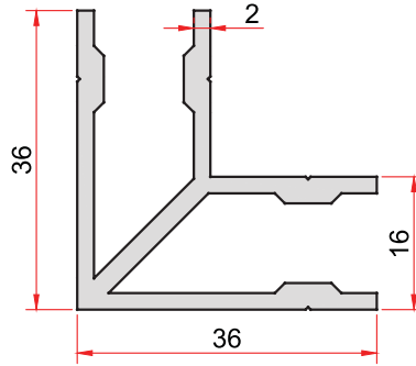
KOD-CODE 840 TEORİK AĞIRLIK THEORETICAL WEIGHT 0,807 Kg/m
