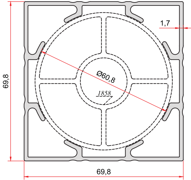
KOD-CODE TEORİK AĞIRLIK THEORETICAL WEIGHT 1898 1,687 Kg/m
