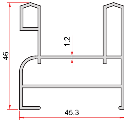
KOD-CODE TEORİK AĞIRLIK THEORETICAL WEIGHT 788 0,802 Kg/m
