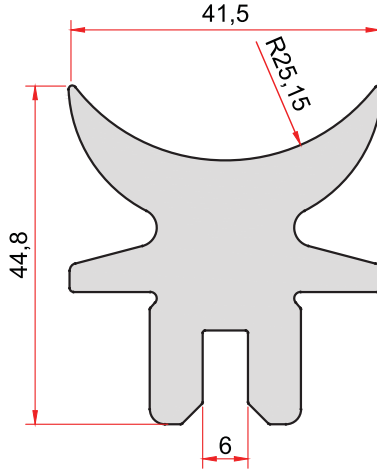
KOD-CODE TEORİK AĞIRLIK THEORETICAL WEIGHT 1857 2,403 Kg/m
