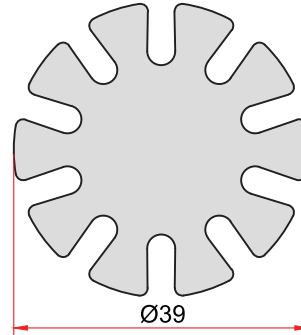
KOD-CODE 5094 TEORİK AĞIRLIK THEORETICAL WEIGHT 2,438 Kg/m
