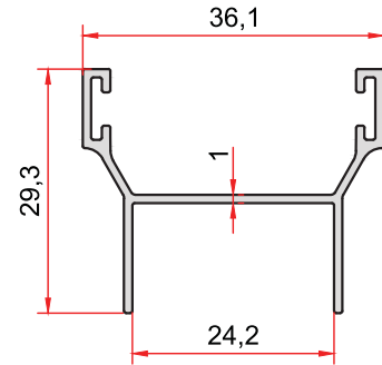
KOD-CODE TEORİK AĞIRLIK 2759 THEORETICAL WEIGHT 0,272 Kg/m
