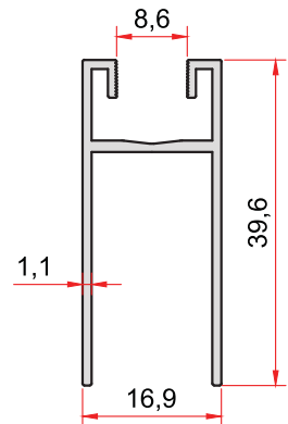
KOD-CODE TEORİK AĞIRLIK 1400 THEORETICAL WEIGHT 0,324 Kg/m
