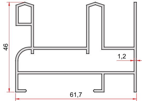
KOD-CODE TEORİK AĞIRLIK THEORETICAL WEIGHT 803 0,999 Kg/m
