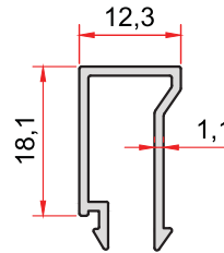
KOD-CODE TEORİK AĞIRLIK SS-302-11 THEORETICAL WEIGHT 0,176 Kg/m
