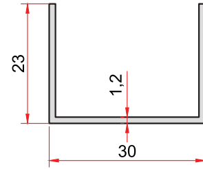
KOD-CODE TEORİK AĞIRLIK 85 THEORETICAL WEIGHT 0,238 Kg/m
