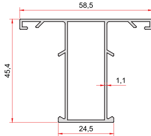
KOD-CODE TEORİK AĞIRLIK 827 THEORETICAL WEIGHT 0,594 Kg/m
