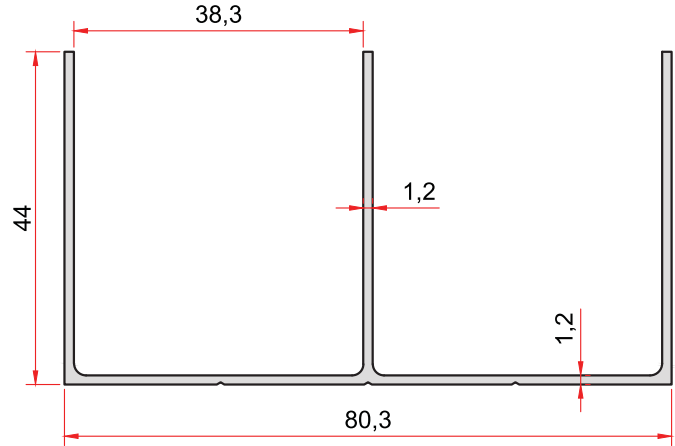
KOD-CODE TEORİK AĞIRLIK THEORETICAL WEIGHT 1424 0,697 Kg/m
