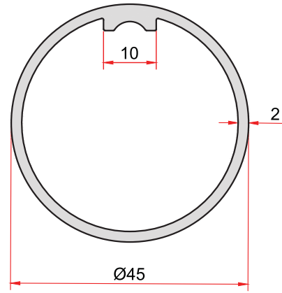
KOD-CODE TEORİK AĞIRLIK THEORETICAL WEIGHT 1969 0,785 Kg/m
