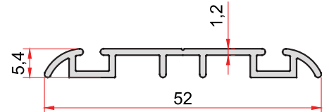
KOD-CODE TEORİK AĞIRLIK THEORETICAL WEIGHT 1372 0,275 Kg/m
