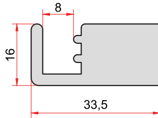
KOD-CODE 1488 TEORİK AĞIRLIK 1,107 Kg/m THEORETICAL WEIGHT
