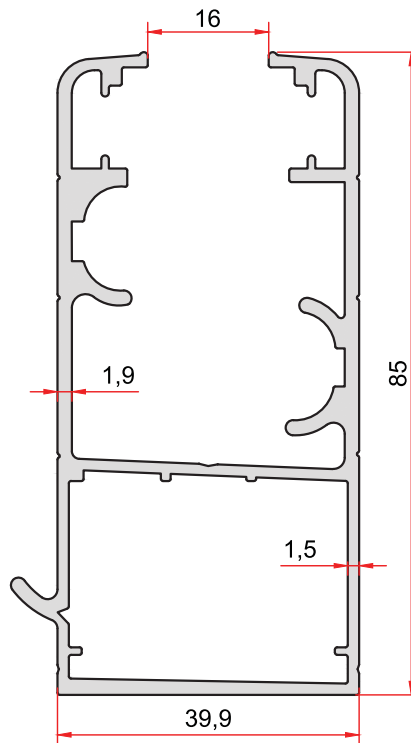
KOD-CODE TEORİK AĞIRLIK 2729 THEORETICAL WEIGHT 1,585 Kg/m
