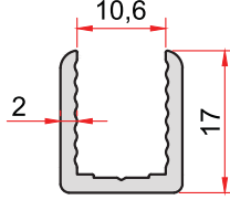
KOD-CODE TEORİK AĞIRLIK 5002 THEORETICAL WEIGHT 0,221 Kg/m
