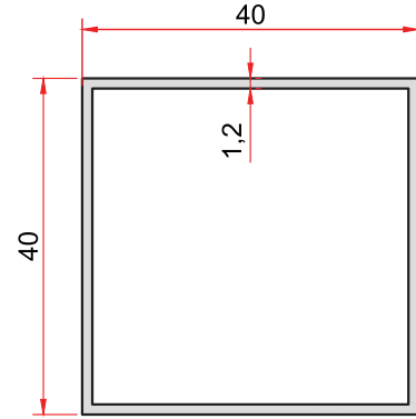
KOD-CODE TEORİK AĞIRLIK THEORETICAL WEIGHT 56 0,502 Kg/m
