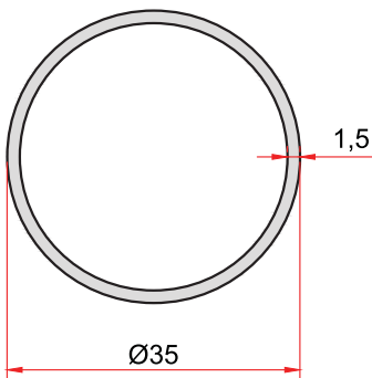
KOD-CODE TEORİK AĞIRLIK 5036 THEORETICAL WEIGHT 0,426 Kg/m
