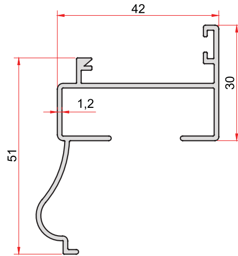
KOD-CODE TEORİK AĞIRLIK THEORETICAL WEIGHT 783 0,535 Kg/m
