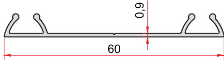
KOD-CODE TEORİK AĞIRLIK THEORETICAL WEIGHT 1450 0,224 Kg/m
