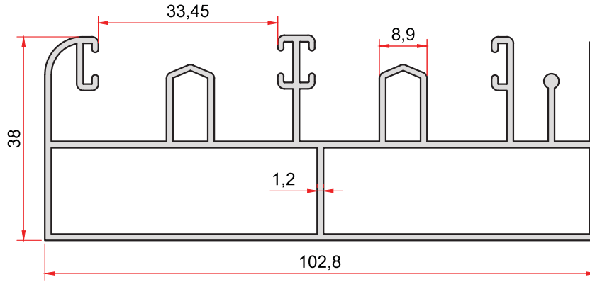
KOD-CODE TEORİK AĞIRLIK 873 THEORETICAL WEIGHT 1,471 Kg/m
