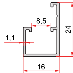
KOD-CODE TEORİK AĞIRLIK 5080 THEORETICAL WEIGHT 0,180 Kg/m
