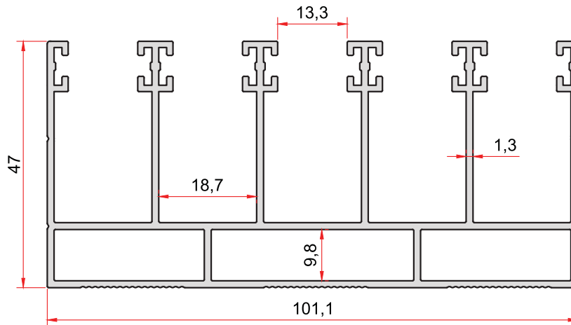
KOD-CODE TEORİK AĞIRLIK 2617 THEORETICAL WEIGHT 1,847 Kg/m
