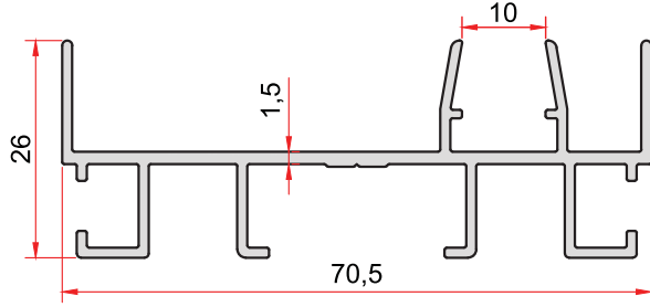
KOD-CODE TEORİK AĞIRLIK 1022 THEORETICAL WEIGHT 0,705 Kg/m
