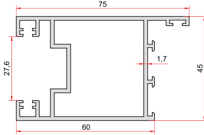
KOD-CODE TEORİK AĞIRLIK 807 THEORETICAL WEIGHT 1,280 Kg/m
