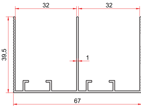
KOD-CODE TEORİK AĞIRLIK THEORETICAL WEIGHT 1502 0,545 Kg/m
