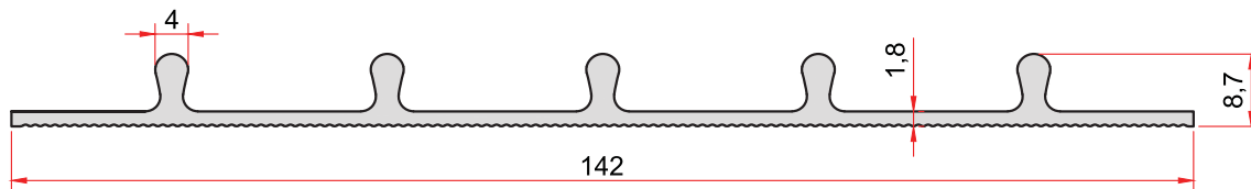
KOD-CODE TEORİK AĞIRLIK THEORETICAL WEIGHT 2384 0,955 Kg/m
