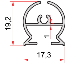
KOD-CODE 1753 TEORİK AĞIRLIK THEORETICAL WEIGHT 0,219 Kg/m
