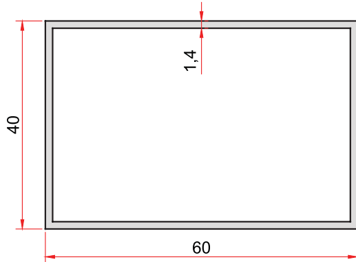
KOD-CODE TEORİK AĞIRLIK THEORETICAL WEIGHT 24 0,734 Kg/m
