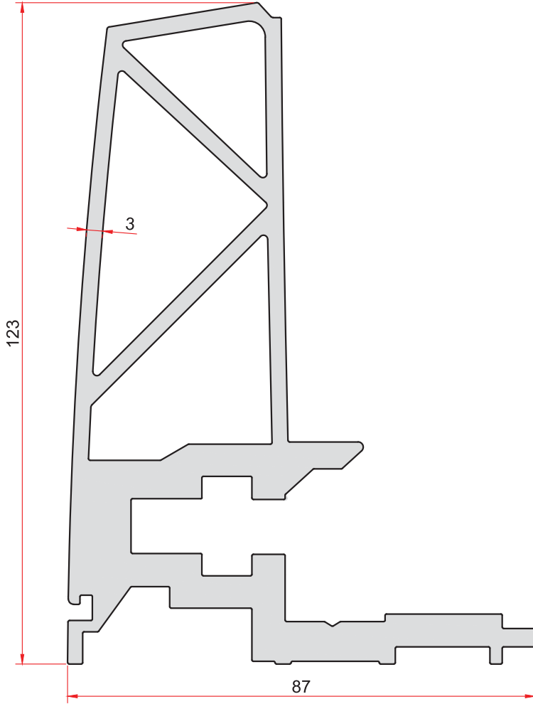
KOD-CODE TEORİK AĞIRLIK 1995 THEORETICAL WEIGHT 5,581 Kg/m
