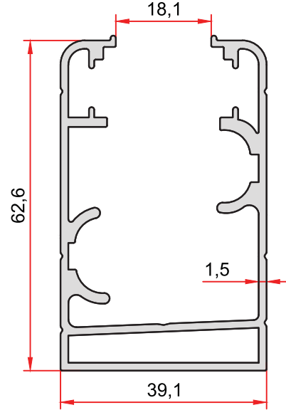
KOD-CODE 2621 TEORİK AĞIRLIK THEORETICAL WEIGHT 1,169 Kg/m
