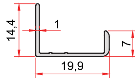
KOD-CODE 778 TEORİK AĞIRLIK THEORETICAL WEIGHT 0,103 Kg/m
