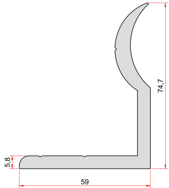
KOD-CODE TEORİK AĞIRLIK THEORETICAL WEIGHT 1864 2,047 Kg/m
