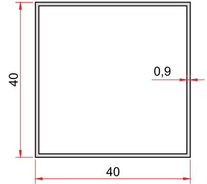
KOD-CODE 1438 TEORİK AĞIRLIK THEORETICAL WEIGHT 0,381 Kg/m
