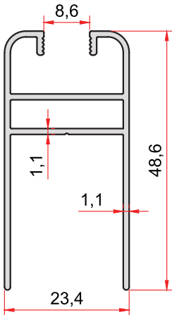
KOD-CODE TEORİK AĞIRLIK 1360 THEORETICAL WEIGHT 0,464 Kg/m
