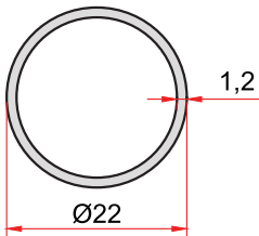
KOD-CODE 1987 TEORİK AĞIRLIK THEORETICAL WEIGHT 0,211 Kg/m
