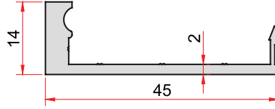
KOD-CODE TEORİK AĞIRLIK 4011 THEORETICAL WEIGHT 0,402 Kg/m
