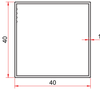
KOD-CODE 773 TEORİK AĞIRLIK THEORETICAL WEIGHT 0,421 Kg/m
