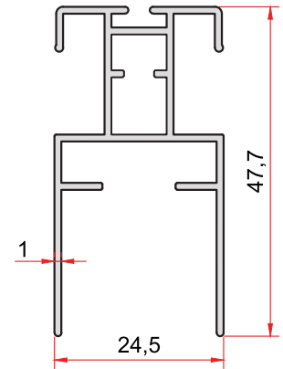
KOD-CODE 1306 TEORİK AĞIRLIK THEORETICAL WEIGHT 0,459 Kg/m
