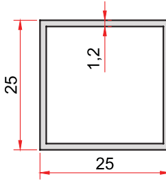
KOD-CODE TEORİK AĞIRLIK 33 THEORETICAL WEIGHT 0,308 Kg/m
