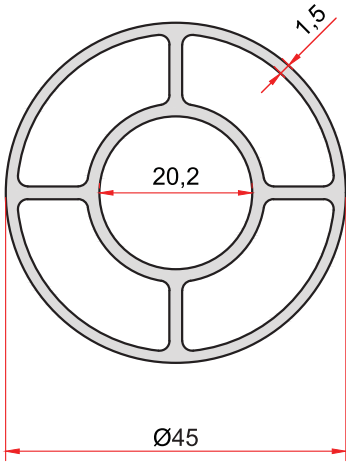
KOD-CODE TEORİK AĞIRLIK 5028 THEORETICAL WEIGHT 1,053 Kg/m
