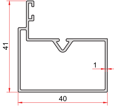
KOD-CODE 2296 TEORİK AĞIRLIK THEORETICAL WEIGHT 0,448 Kg/m
