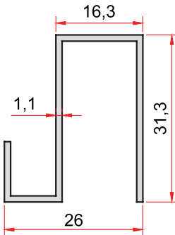
KOD-CODE 1366 TEORİK AĞIRLIK THEORETICAL WEIGHT 0,300 Kg/m
