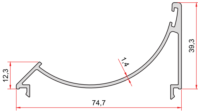
KOD-CODE TEORİK AĞIRLIK THEORETICAL WEIGHT 1202 0,621 Kg/m
