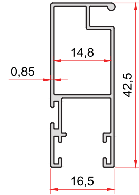
KOD-CODE 1310 TEORİK AĞIRLIK THEORETICAL WEIGHT 0,335 Kg/m
