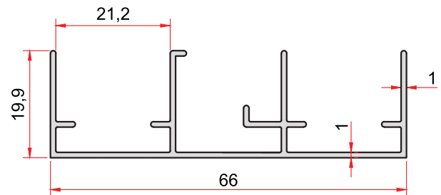
KOD-CODE TEORİK AĞIRLIK THEORETICAL WEIGHT 1453 0,451 Kg/m
