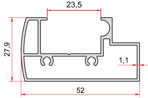
KOD-CODE TEORİK AĞIRLIK 1762 THEORETICAL WEIGHT 0,640 Kg/m
