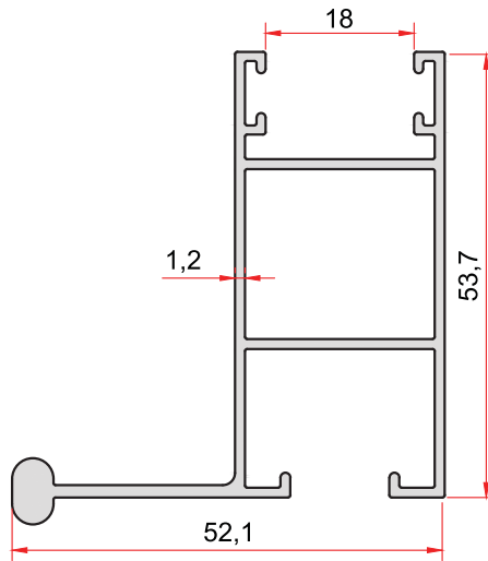
KOD-CODE 1013 TEORİK AĞIRLIK THEORETICAL WEIGHT 0,775 Kg/m
