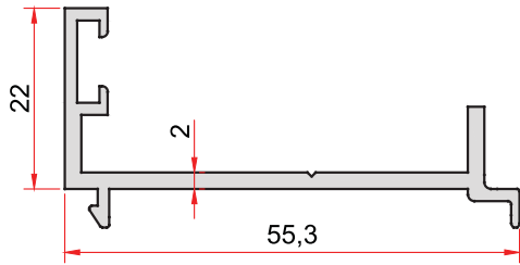
KOD-CODE 848 TEORİK AĞIRLIK THEORETICAL WEIGHT 0,502 Kg/m
