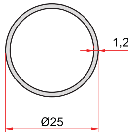
KOD-CODE 5035 TEORİK AĞIRLIK THEORETICAL WEIGHT 0,243 Kg/m
