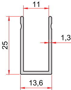
KOD-CODE TEORİK AĞIRLIK 5015 THEORETICAL WEIGHT 0,210 Kg/m
