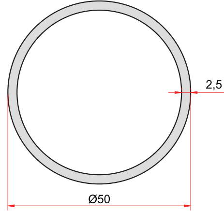
KOD-CODE TEORİK AĞIRLIK THEORETICAL WEIGHT 1923 1,007 Kg/m
