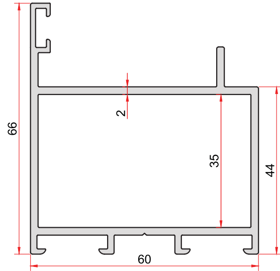
KOD-CODE TEORİK AĞIRLIK 1170 THEORETICAL WEIGHT 1,336 Kg/m
