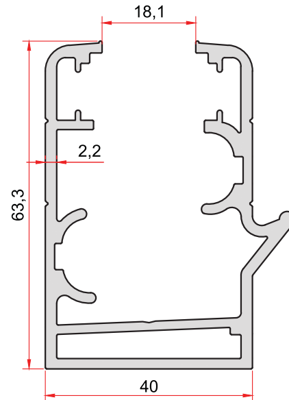
KOD-CODE 2272 TEORİK AĞIRLIK 1,545 Kg/m THEORETICAL WEIGHT
