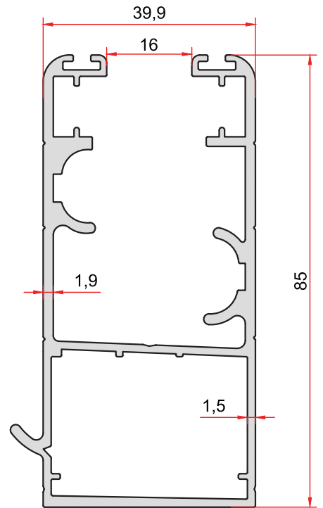
KOD-CODE TEORİK AĞIRLIK THEORETICAL WEIGHT 2728 1,596 Kg/m
