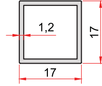
KOD-CODE 1985 TEORİK AĞIRLIK 0,203 Kg/m THEORETICAL WEIGHT
