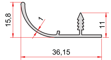
KOD-CODE 1484 TEORİK AĞIRLIK THEORETICAL WEIGHT 0,211 Kg/m
