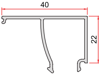
KOD-CODE TEORİK AĞIRLIK CC-1400-13 THEORETICAL WEIGHT 0,341 Kg/m
