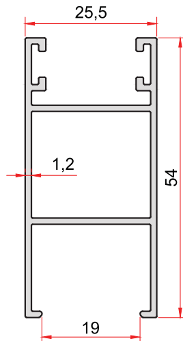
KOD-CODE TEORİK AĞIRLIK 1021 THEORETICAL WEIGHT 0,569 Kg/m
