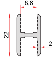
KOD-CODE TEORİK AĞIRLIK 5003 THEORETICAL WEIGHT 0,270 Kg/m
