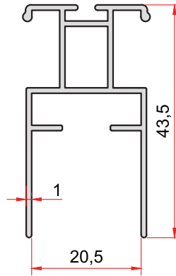
KOD-CODE 1308 TEORİK AĞIRLIK THEORETICAL WEIGHT 0,413 Kg/m
