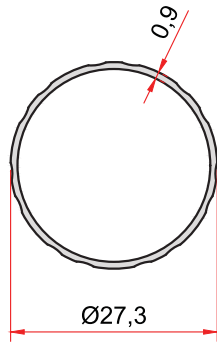
KOD-CODE 4022 TEORİK AĞIRLIK THEORETICAL WEIGHT 0,189 Kg/m
