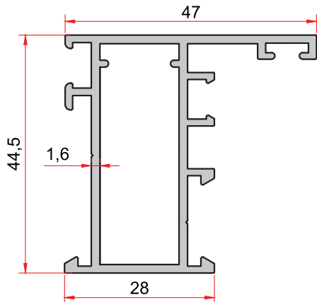
KOD-CODE TEORİK AĞIRLIK THEORETICAL WEIGHT 1089 0,826 Kg/m
