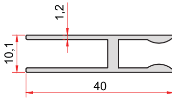
KOD-CODE TEORİK AĞIRLIK 869 0,340 Kg/m
