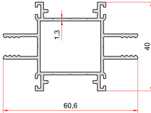
KOD-CODE TEORİK AĞIRLIK THEORETICAL WEIGHT AO-1011-13 0,805 Kg/m
