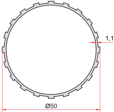
KOD-CODE TEORİK AĞIRLIK THEORETICAL WEIGHT 1901 0,586 Kg/m
