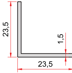
KOD-CODE 135 TEORİK AĞIRLIK THEORETICAL WEIGHT 0,184 Kg/m
