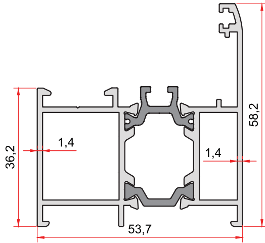
KOD-CODE TEORİK AĞIRLIK İD-101-14 THEORETICAL WEIGHT 1,214 Kg/m
