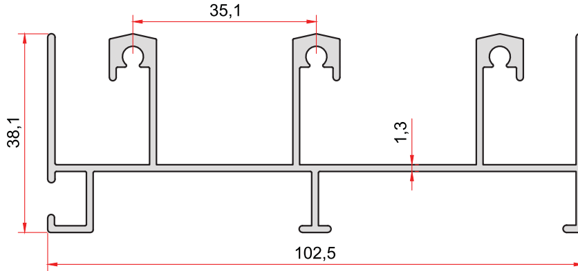
KOD-CODE TEORİK AĞIRLIK THEORETICAL WEIGHT 1079 1,288 Kg/m
