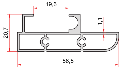
KOD-CODE TEORİK AĞIRLIK 1786 THEORETICAL WEIGHT 0,594 Kg/m
