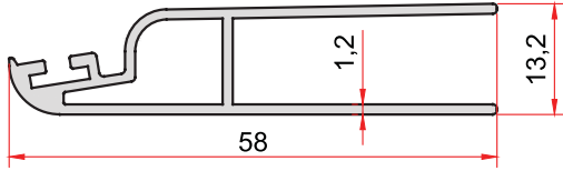
KOD-CODE 798 TEORİK AĞIRLIK THEORETICAL WEIGHT 0,465 Kg/m
