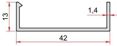
KOD-CODE TEORİK AĞIRLIK 4003 THEORETICAL WEIGHT 0,248 Kg/m
