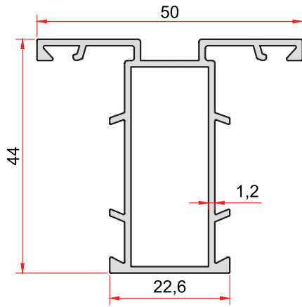
KOD-CODE TEORİK AĞIRLIK THEORETICAL WEIGHT 1083 0,626 Kg/m
