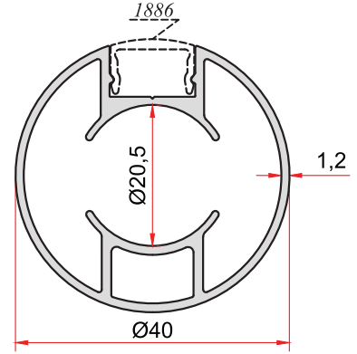
KOD-CODE 1890 TEORİK AĞIRLIK THEORETICAL WEIGHT 0,645 Kg/m
