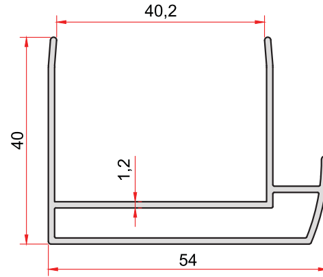
KOD-CODE 2619 TEORİK AĞIRLIK THEORETICAL WEIGHT 0,610 Kg/m
