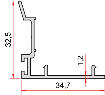
KOD-CODE TEORİK AĞIRLIK 819 THEORETICAL WEIGHT 0,283 Kg/m
