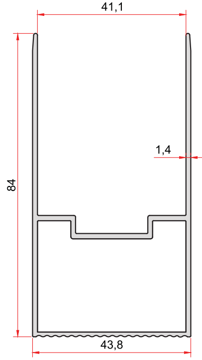
KOD-CODE TEORİK AĞIRLIK 2274 THEORETICAL WEIGHT 0,929 Kg/m
