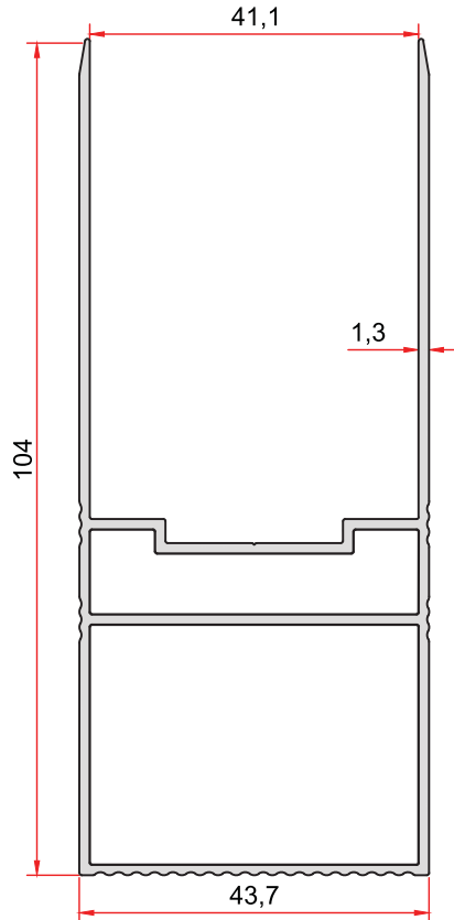
KOD-CODE TEORİK AĞIRLIK 2663 THEORETICAL WEIGHT 1,150 Kg/m
