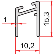
KOD-CODE 2391 TEORİK AĞIRLIK THEORETICAL WEIGHT 0,116 Kg/m
