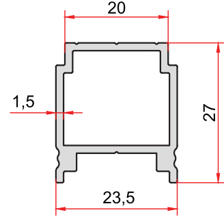
KOD-CODE 2678 TEORİK AĞIRLIK THEORETICAL WEIGHT 0,421 Kg/m
