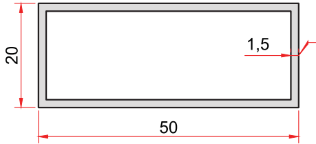
KOD-CODE TEORİK AĞIRLIK THEORETICAL WEIGHT 115 0,542 Kg/m
