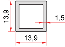
KOD-CODE 1960 TEORİK AĞIRLIK 0,199 Kg/m THEORETICAL WEIGHT
