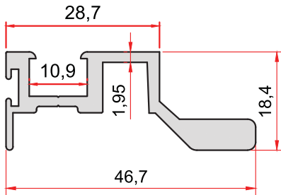
KOD-CODE 1368 TEORİK AĞIRLIK THEORETICAL WEIGHT 0,637 Kg/m
