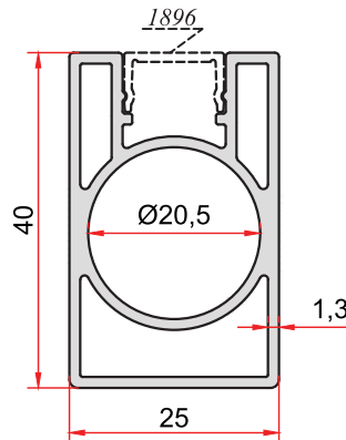
KOD-CODE 5049 TEORİK AĞIRLIK 0,723 Kg/m THEORETICAL WEIGHT
