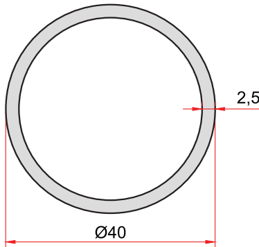
KOD-CODE TEORİK AĞIRLIK 1900 THEORETICAL WEIGHT 0,793 Kg/m
