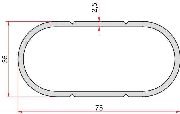
KOD-CODE TEORİK AĞIRLIK THEORETICAL WEIGHT 1419 1,212 Kg/m
