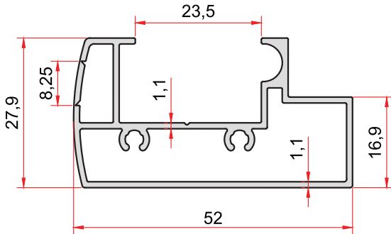
KOD-CODE TEORİK AĞIRLIK 1787 THEORETICAL WEIGHT 0,632 Kg/m
