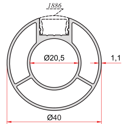
KOD-CODE 1931 TEORİK AĞIRLIK THEORETICAL WEIGHT 0,672 Kg/m
