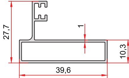
KOD-CODE TEORİK AĞIRLIK 2763 THEORETICAL WEIGHT 0,356 Kg/m
