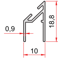
KOD-CODE 2264 TEORİK AĞIRLIK THEORETICAL WEIGHT 0,113 Kg/m
