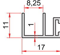
KOD-CODE 2625 TEORİK AĞIRLIK THEORETICAL WEIGHT 0,135 Kg/m
