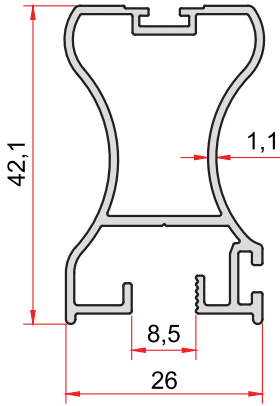
KOD-CODE 1363 TEORİK AĞIRLIK THEORETICAL WEIGHT 0,494 Kg/m
