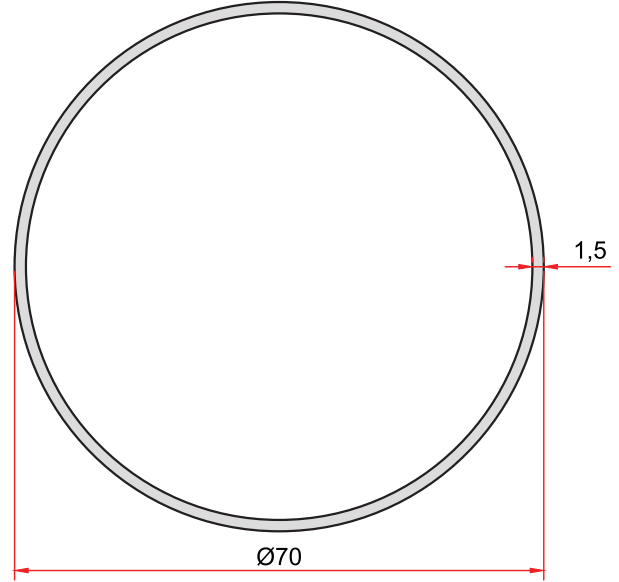
KOD-CODE TEORİK AĞIRLIK THEORETICAL WEIGHT 5050 0,872 Kg/m
