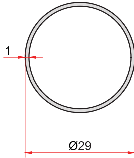
KOD-CODE 2220 TEORİK AĞIRLIK THEORETICAL WEIGHT 0,237 Kg/m
