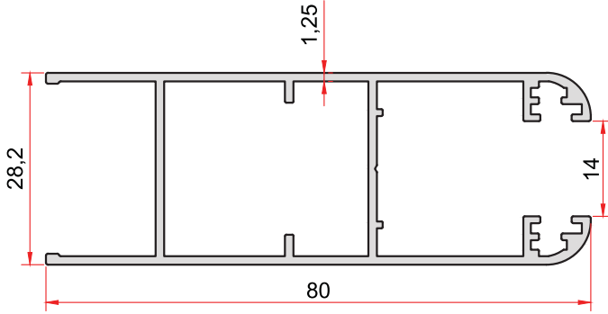
KOD-CODE TEORİK AĞIRLIK 1135 THEORETICAL WEIGHT 0,848 Kg/m
