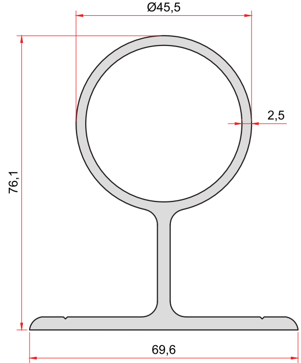
KOD-CODE TEORİK AĞIRLIK THEORETICAL WEIGHT 1868 1,798 Kg/m
