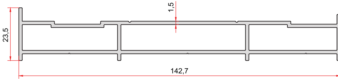
KOD-CODE 2672 TEORİK AĞIRLIK THEORETICAL WEIGHT 1,439 Kg/m
