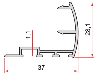
KOD-CODE TEORİK AĞIRLIK THEORETICAL WEIGHT 1068 0,286 Kg/m
