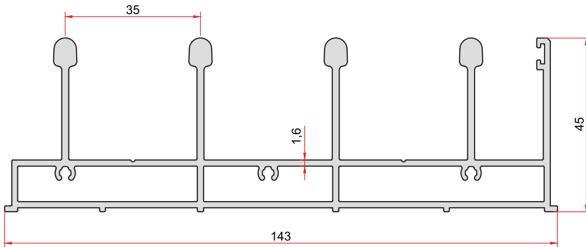
KOD-CODE 2669 TEORİK AĞIRLIK THEORETICAL WEIGHT 2,538 Kg/m
