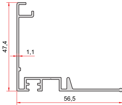
KOD-CODE TEORİK AĞIRLIK THEORETICAL WEIGHT MD-102-11 0,461 Kg/m
