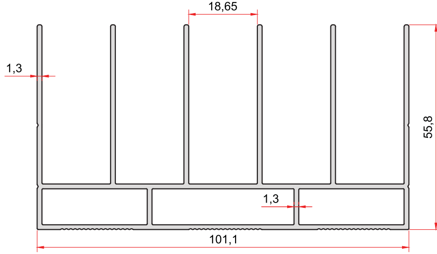
KOD-CODE TEORİK AĞIRLIK THEORETICAL WEIGHT 2438 1,741 Kg/m
