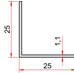
KOD-CODE 15 TEORİK AĞIRLIK THEORETICAL WEIGHT 0,146 Kg/m
