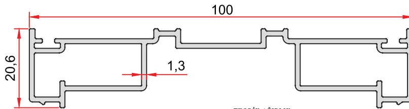
KOD-CODE TEORİK AĞIRLIK THEORETICAL WEIGHT AO-1012-13 0,874 Kg/m
