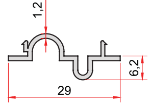
KOD-CODE TEORİK AĞIRLIK 818 THEORETICAL WEIGHT 0,167 Kg/m
