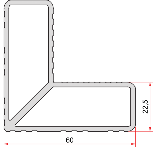
KOD-CODE TEORİK AĞIRLIK THEORETICAL WEIGHT KT-225-00 1,508 Kg/m
