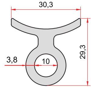
KOD-CODE 5032 TEORİK AĞIRLIK THEORETICAL WEIGHT 0,788 Kg/m
