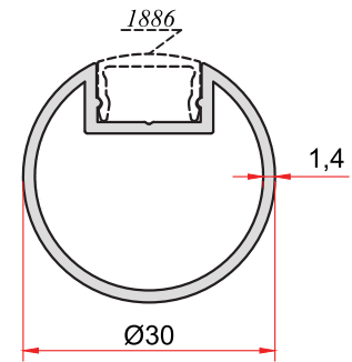
KOD-CODE TEORİK AĞIRLIK 1991 THEORETICAL WEIGHT 0,391 Kg/m
