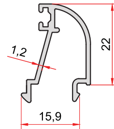
KOD-CODE TEORİK AĞIRLIK İS-804-12 THEORETICAL WEIGHT 0,243 Kg/m
