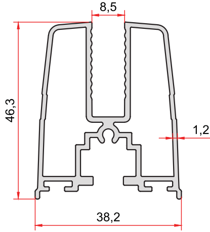
KOD-CODE 2753 TEORİK AĞIRLIK THEORETICAL WEIGHT 0,888 Kg/m
