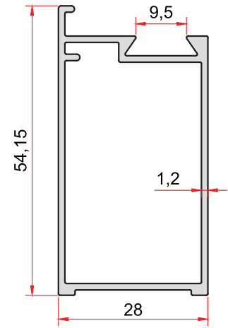
KOD-CODE 1032 TEORİK AĞIRLIK THEORETICAL WEIGHT 0,575 Kg/m
