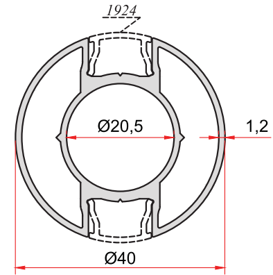
KOD-CODE 1925 TEORİK AĞIRLIK THEORETICAL WEIGHT 0,721 Kg/m
