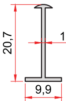
KOD-CODE TEORİK AĞIRLIK THEORETICAL WEIGHT 1432 0,086 Kg/m
