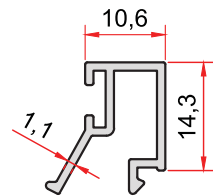
KOD-CODE TEORİK AĞIRLIK THEORETICAL WEIGHT SS-301-11 0,165 Kg/m
