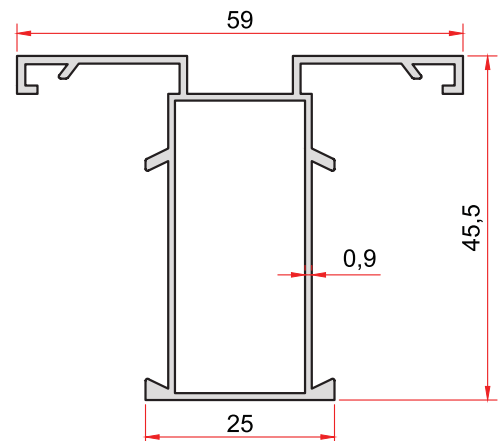
KOD-CODE TEORİK AĞIRLIK 862 THEORETICAL WEIGHT 0,537 Kg/m
