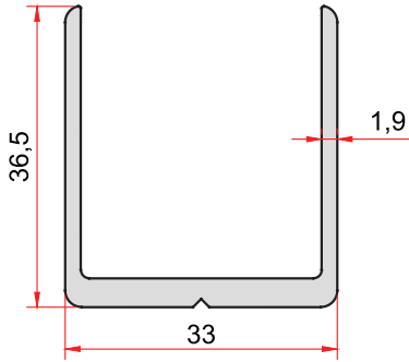
KOD-CODE 842 TEORİK AĞIRLIK THEORETICAL WEIGHT 0,640 Kg/m
