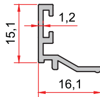
KOD-CODE TEORİK AĞIRLIK 879 THEORETICAL WEIGHT 0,140 Kg/m
