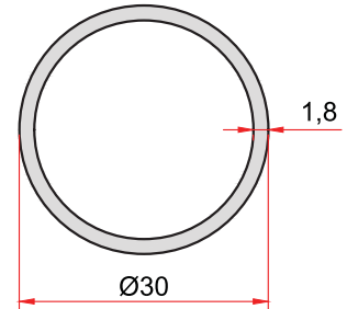
KOD-CODE TEORİK AĞIRLIK 1911 THEORETICAL WEIGHT 0,429 Kg/m
