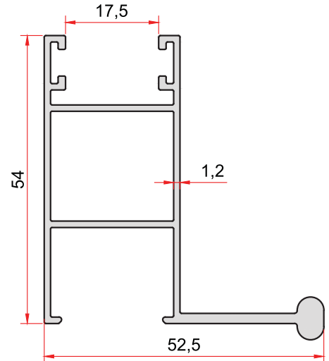
KOD-CODE 1014 TEORİK AĞIRLIK THEORETICAL WEIGHT 0,776 Kg/m
