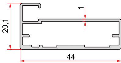
KOD-CODE 1460 TEORİK AĞIRLIK 0,410 Kg/m THEORETICAL WEIGHT
