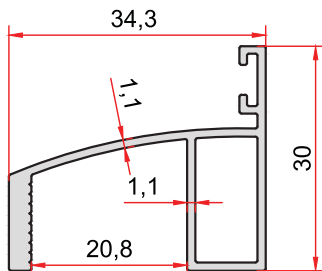
KOD-CODE TEORİK AĞIRLIK 2750 THEORETICAL WEIGHT 0,383 Kg/m
