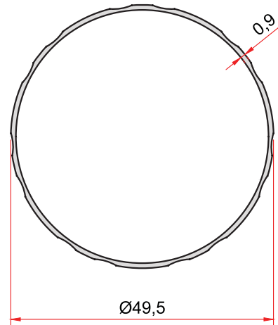
KOD-CODE 4021 TEORİK AĞIRLIK THEORETICAL WEIGHT 0,356 Kg/m
