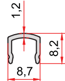
KOD-CODE TEORİK AĞIRLIK 5101 THEORETICAL WEIGHT 0,062 Kg/m
