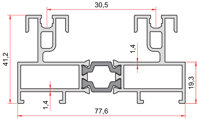
KOD-CODE TEORİK AĞIRLIK İS-101-14 THEORETICAL WEIGHT 1,572 Kg/m
