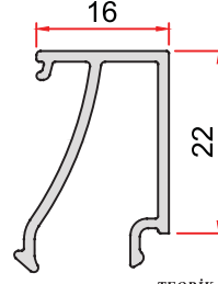
KOD-CODE TEORİK AĞIRLIK CC-1160-13 THEORETICAL WEIGHT 0,260 Kg/m
