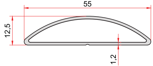
KOD-CODE 5069 TEORİK AĞIRLIK THEORETICAL WEIGHT 0,372 Kg/m
