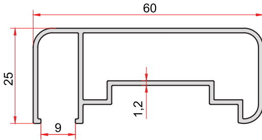
KOD-CODE 5079 TEORİK AĞIRLIK THEORETICAL WEIGHT 0,607 Kg/m
