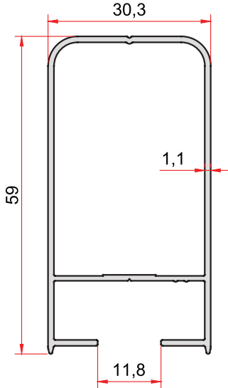
KOD-CODE 769 TEORİK AĞIRLIK THEORETICAL WEIGHT 0,543 Kg/m
