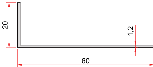
KOD-CODE TEORİK AĞIRLIK THEORETICAL WEIGHT 18 0,257 Kg/m
