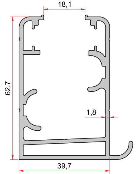
KOD-CODE TEORİK AĞIRLIK THEORETICAL WEIGHT 2450 1,378 Kg/m
