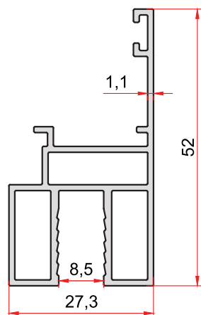
KOD-CODE 7043 TEORİK AĞIRLIK 0,583 Kg/m THEORETICAL WEIGHT
