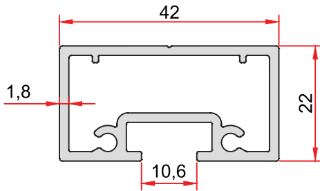
KOD-CODE TEORİK AĞIRLIK THEORETICAL WEIGHT AO-1027-18 0,736 Kg/m
