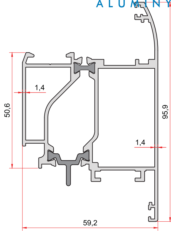
KOD-CODE TEORİK AĞIRLIK İD-601-15 THEORETICAL WEIGHT 1,763 Kg/m
