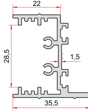
KOD-CODE 2632 TEORİK AĞIRLIK THEORETICAL WEIGHT 0,656 Kg/m
