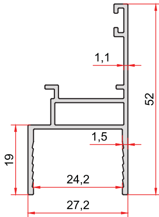
KOD-CODE 2755 TEORİK AĞIRLIK 0,434 Kg/m THEORETICAL WEIGHT
