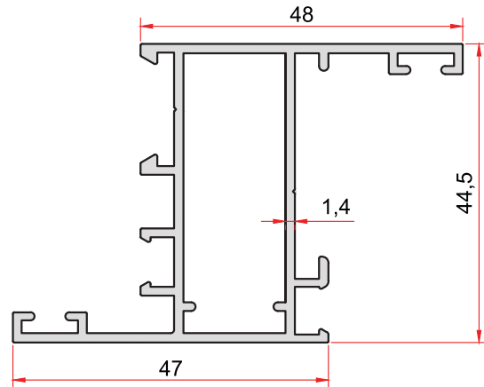
KOD-CODE TEORİK AĞIRLIK 1086 THEORETICAL WEIGHT 0,859 Kg/m
