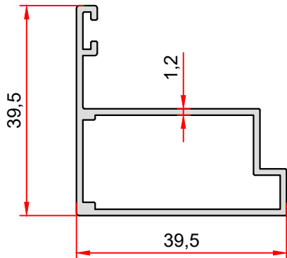
KOD-CODE TEORİK AĞIRLIK 2660 THEORETICAL WEIGHT 0,472 Kg/m
