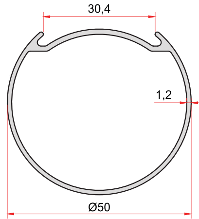
KOD-CODE TEORİK AĞIRLIK 5030 THEORETICAL WEIGHT 0,543 Kg/m
