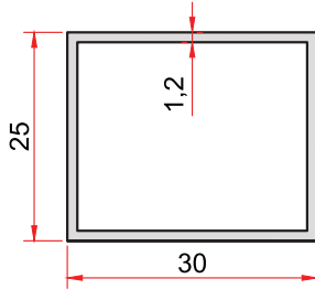
KOD-CODE TEORİK AĞIRLIK 32 THEORETICAL WEIGHT 0,341 Kg/m
