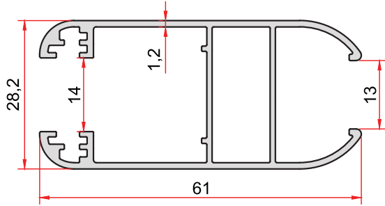
KOD-CODE TEORİK AĞIRLIK THEORETICAL WEIGHT 784 0,685 Kg/m
