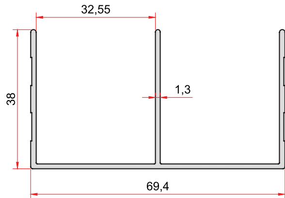
KOD-CODE TEORİK AĞIRLIK THEORETICAL WEIGHT 1358 0,641 Kg/m
