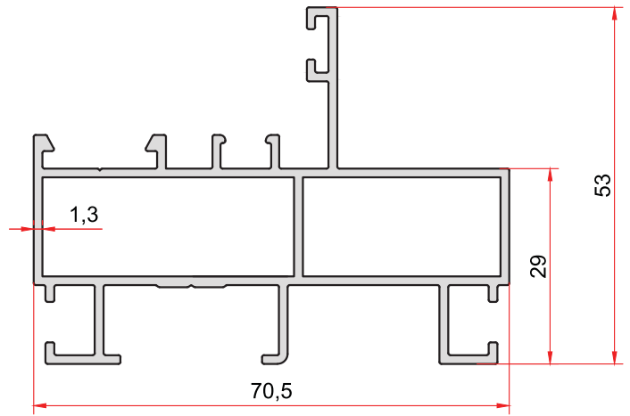
KOD-CODE TEORİK AĞIRLIK 7034 THEORETICAL WEIGHT 1,085 Kg/m
