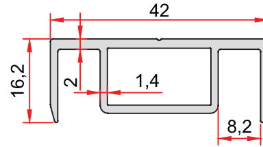
KOD-CODE TEORİK AĞIRLIK THEORETICAL WEIGHT AO-1028-14 0,491 Kg/m
