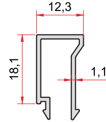
KOD-CODE TEORİK AĞIRLIK THEORETICAL WEIGHT SS-302-11 0,176 Kg/m
