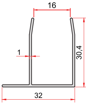
KOD-CODE 1767 TEORİK AĞIRLIK THEORETICAL WEIGHT 0,243 Kg/m
