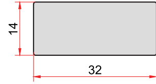
KOD-CODE TEORİK AĞIRLIK THEORETICAL WEIGHT 144 1,209 Kg/m
