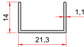
KOD-CODE TEORİK AĞIRLIK THEORETICAL WEIGHT 1388 0,140 Kg/m
