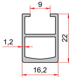
KOD-CODE TEORİK AĞIRLIK 1950 THEORETICAL WEIGHT 0,273 Kg/m
