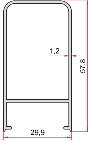
KOD-CODE 875 TEORİK AĞIRLIK THEORETICAL WEIGHT 0,551 Kg/m
