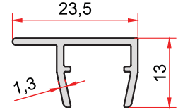
KOD-CODE 1028 TEORİK AĞIRLIK THEORETICAL WEIGHT 0,171 Kg/m
