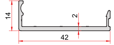
KOD-CODE TEORİK AĞIRLIK 4012 THEORETICAL WEIGHT 0,292 Kg/m
