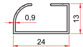
KOD-CODE 779 TEORİK AĞIRLIK THEORETICAL WEIGHT 0,143 Kg/m
