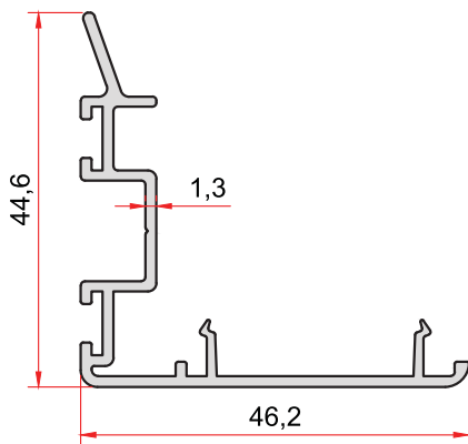
KOD-CODE TEORİK AĞIRLIK SS-404-13 THEORETICAL WEIGHT 0,468 Kg/m
