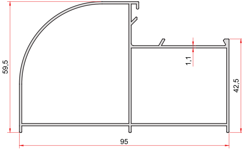
KOD-CODE TEORİK AĞIRLIK 806 THEORETICAL WEIGHT 1,023 Kg/m
