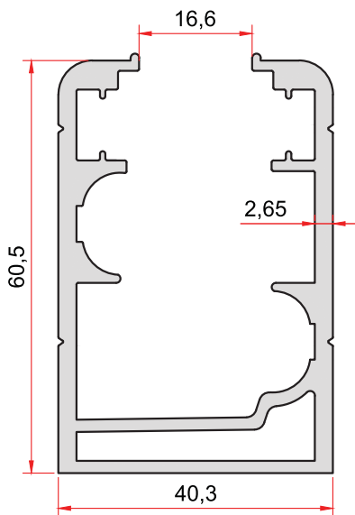
KOD-CODE TEORİK AĞIRLIK 2263 THEORETICAL WEIGHT 1,569 Kg/m
