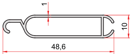
KOD-CODE TEORİK AĞIRLIK 2305 THEORETICAL WEIGHT 0,297 Kg/m
