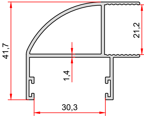
KOD-CODE TEORİK AĞIRLIK 2668 THEORETICAL WEIGHT 0,621 Kg/m
