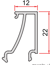
KOD-CODE TEORİK AĞIRLIK CC-1120-13 THEORETICAL WEIGHT 0,254 Kg/m
