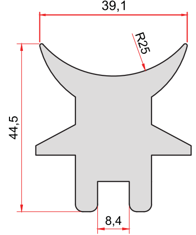
KOD-CODE TEORİK AĞIRLIK THEORETICAL WEIGHT 1966 2,397 Kg/m
