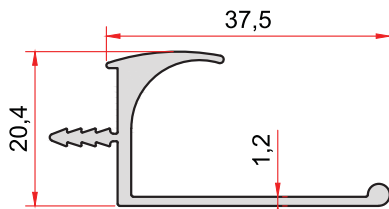
KOD-CODE 1498 TEORİK AĞIRLIK THEORETICAL WEIGHT 0,377 Kg/m
