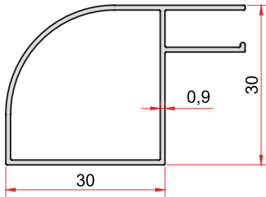
KOD-CODE 772 TEORİK AĞIRLIK THEORETICAL WEIGHT 0,337 Kg/m
