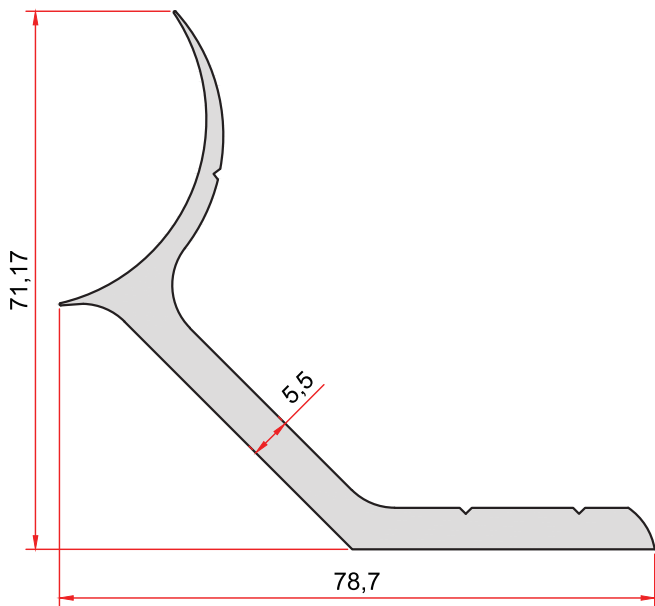
KOD-CODE TEORİK AĞIRLIK THEORETICAL WEIGHT 1869 1,528 Kg/m
