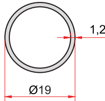
KOD-CODE 1880 TEORİK AĞIRLIK THEORETICAL WEIGHT 0,181 Kg/m
