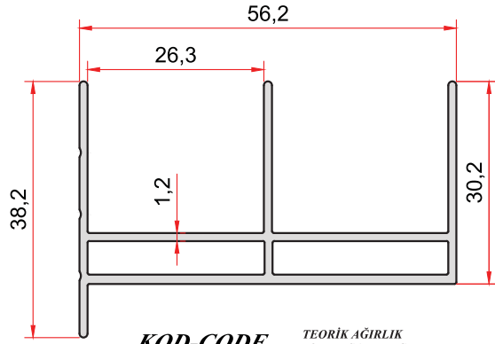
KOD-CODE 99 TEORİK AĞIRLIK THEORETICAL WEIGHT 0,685 Kg/m
