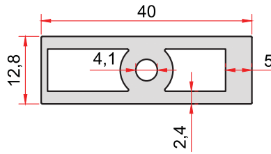
KOD-CODE 1493 TEORİK AĞIRLIK THEORETICAL WEIGHT 0,807 Kg/m
