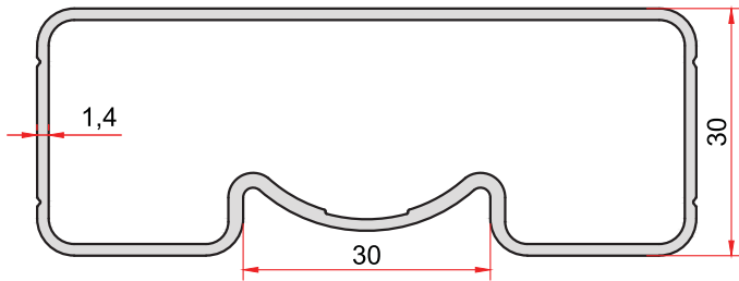
KOD-CODE TEORİK AĞIRLIK THEORETICAL WEIGHT 5034 0,877 Kg/m
