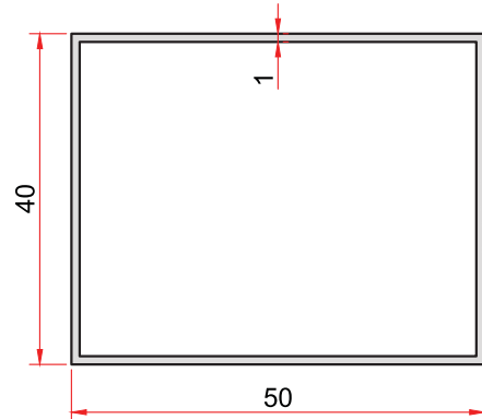
KOD-CODE TEORİK AĞIRLIK THEORETICAL WEIGHT 35 0,475 Kg/m
