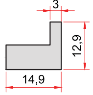
KOD-CODE 1409 TEORİK AĞIRLIK THEORETICAL WEIGHT 0,319 Kg/m
