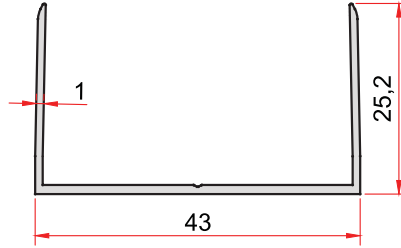
KOD-CODE TEORİK AĞIRLIK 2297 THEORETICAL WEIGHT 0,265 Kg/m
