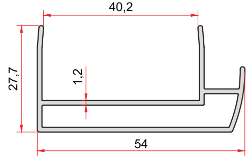
KOD-CODE 2392 TEORİK AĞIRLIK THEORETICAL WEIGHT 0,532 Kg/m
