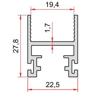
KOD-CODE 109 TEORİK AĞIRLIK THEORETICAL WEIGHT 0,413 Kg/m
