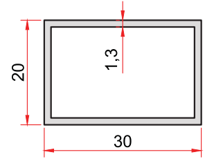
KOD-CODE TEORİK AĞIRLIK 49 THEORETICAL WEIGHT 0,332 Kg/m
