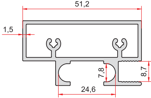
KOD-CODE TEORİK AĞIRLIK THEORETICAL WEIGHT 1790 0,885 Kg/m
