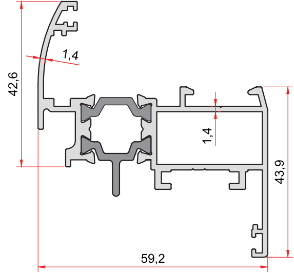
KOD-CODE TEORİK AĞIRLIK İD-401-14 THEORETICAL WEIGHT 1,197 Kg/m
