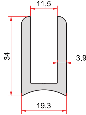
KOD-CODE 1986 TEORİK AĞIRLIK THEORETICAL WEIGHT 0,780 Kg/m
