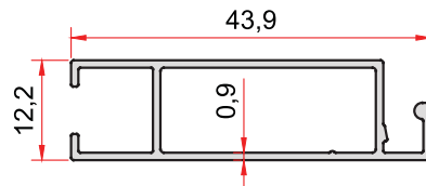
KOD-CODE TEORİK AĞIRLIK THEORETICAL WEIGHT 768 0,283 Kg/m
