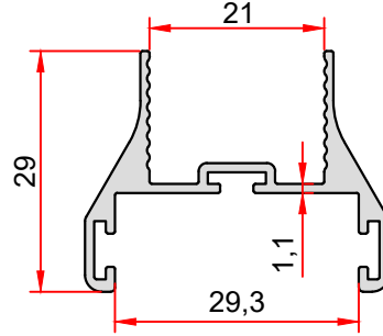
KOD-CODE TEORİK AĞIRLIK 2656 THEORETICAL WEIGHT 0,423 Kg/m
