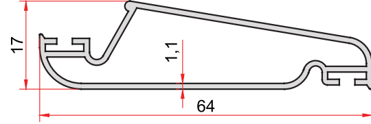
KOD-CODE 797 TEORİK AĞIRLIK THEORETICAL WEIGHT 0,486 Kg/m
