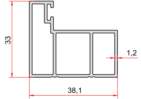
KOD-CODE 2731 TEORİK AĞIRLIK 0,578 Kg/m THEORETICAL WEIGHT
