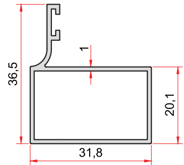
KOD-CODE TEORİK AĞIRLIK 2262 THEORETICAL WEIGHT 0,359 Kg/m
