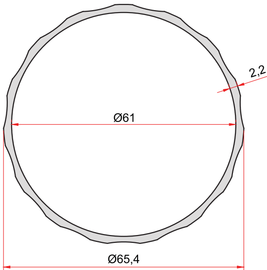
KOD-CODE TEORİK AĞIRLIK THEORETICAL WEIGHT 1963 1,011 Kg/m
