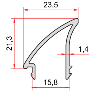
KOD-CODE TEORİK AĞIRLIK 5019 THEORETICAL WEIGHT 0,251 Kg/m
