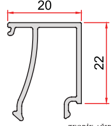
KOD-CODE TEORİK AĞIRLIK CC-1200-13 THEORETICAL WEIGHT 0,270 Kg/m
