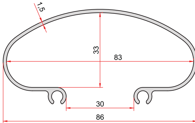
KOD-CODE TEORİK AĞIRLIK 5062 THEORETICAL WEIGHT 0,785 Kg/m
