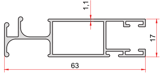
KOD-CODE TEORİK AĞIRLIK 1311 THEORETICAL WEIGHT 0,548 Kg/m
