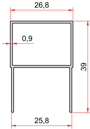
KOD-CODE 1307 TEORİK AĞIRLIK THEORETICAL WEIGHT 0,311 Kg/m
