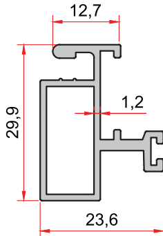
KOD-CODE 1072 TEORİK AĞIRLIK THEORETICAL WEIGHT 0,397 Kg/m
