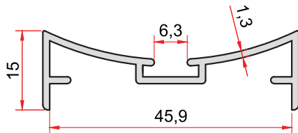
KOD-CODE 878 TEORİK AĞIRLIK THEORETICAL WEIGHT 0,335 Kg/m
