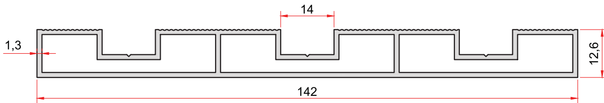
KOD-CODE TEORİK AĞIRLIK THEORETICAL WEIGHT 2383 1,247 Kg/m
