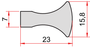
KOD-CODE 1439 TEORİK AĞIRLIK THEORETICAL WEIGHT 0,489 Kg/m
