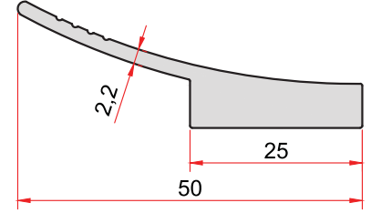
KOD-CODE 1471 TEORİK AĞIRLIK THEORETICAL WEIGHT 0,645 Kg/m
