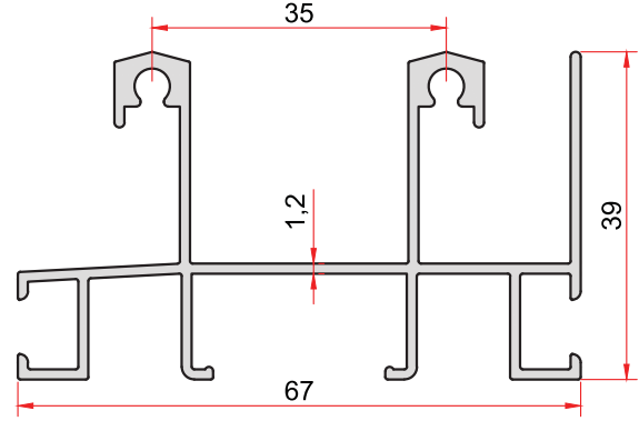
KOD-CODE TEORİK AĞIRLIK 1081 THEORETICAL WEIGHT 0,888 Kg/m
