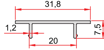
KOD-CODE TEORİK AĞIRLIK THEORETICAL WEIGHT AO-1041-12 0,145 Kg/m
