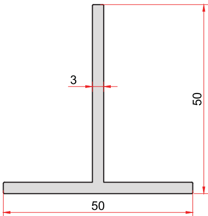
KOD-CODE 80 TEORİK AĞIRLIK THEORETICAL WEIGHT 0,786 Kg/m
