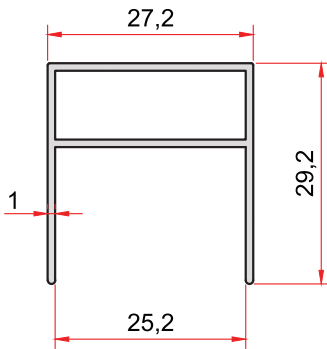
KOD-CODE 1304 TEORİK AĞIRLIK THEORETICAL WEIGHT 0,294 Kg/m
