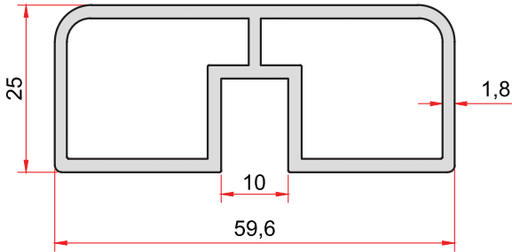
KOD-CODE TEORİK AĞIRLIK 1876 THEORETICAL WEIGHT 1,010 Kg/m
