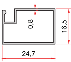
KOD-CODE 1301 TEORİK AĞIRLIK THEORETICAL WEIGHT 0,189 Kg/m
