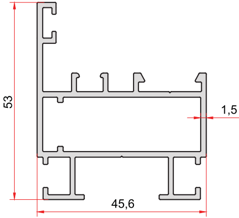
KOD-CODE TEORİK AĞIRLIK 7033 THEORETICAL WEIGHT 0,899 Kg/m
