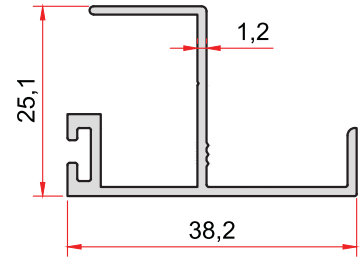
KOD-CODE TEORİK AĞIRLIK THEORETICAL WEIGHT 1404 0,338 Kg/m
