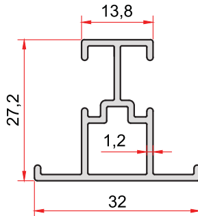
KOD-CODE 1029 TEORİK AĞIRLIK THEORETICAL WEIGHT 0,348 Kg/m
