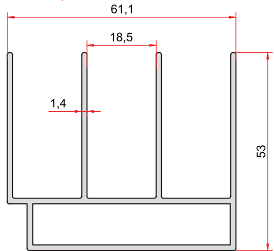
KOD-CODE TEORİK AĞIRLIK 2699 THEORETICAL WEIGHT 1,150 Kg/m
