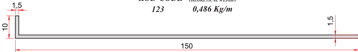
KOD-CODE TEORİK AĞIRLIK THEORETICAL WEIGHT 13 0,645 Kg/m
