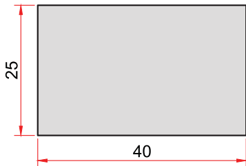
KOD-CODE TEORİK AĞIRLIK THEORETICAL WEIGHT 69 2,700 Kg/m
