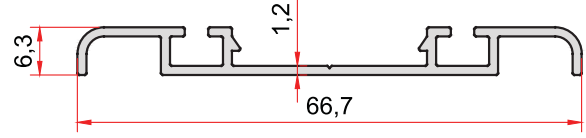
KOD-CODE TEORİK AĞIRLIK THEORETICAL WEIGHT 1355 0,337 Kg/m
