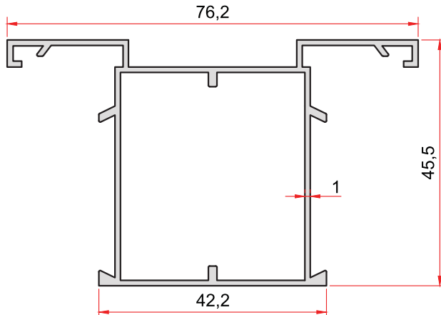
KOD-CODE TEORİK AĞIRLIK 856 THEORETICAL WEIGHT 0,683 Kg/m
