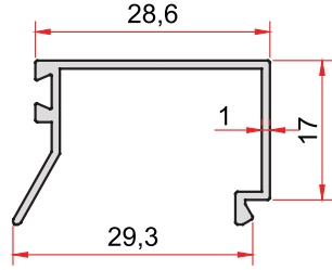
KOD-CODE TEORİK AĞIRLIK 811 0,213 Kg/m
