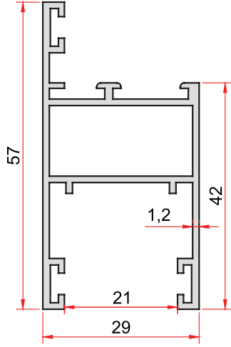
KOD-CODE TEORİK AĞIRLIK 814 THEORETICAL WEIGHT 0,634 Kg/m
