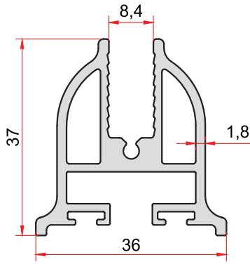
KOD-CODE TEORİK AĞIRLIK THEORETICAL WEIGHT 2269 0,875 Kg/m
