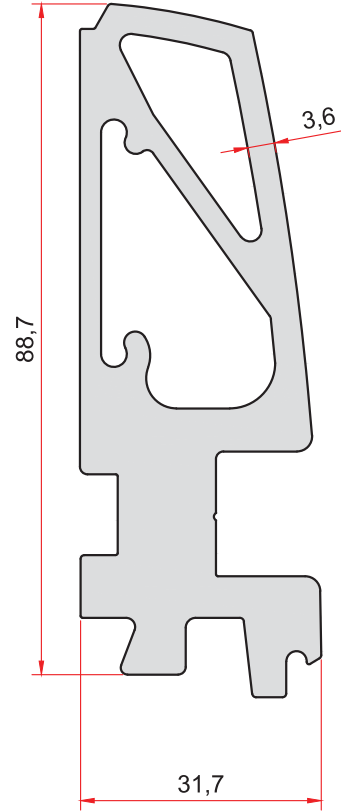
KOD-CODE TEORİK AĞIRLIK THEORETICAL WEIGHT 2276 3,591 Kg/m
