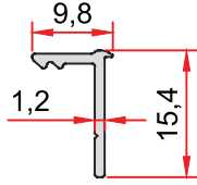
KOD-CODE TEORİK AĞIRLIK THEORETICAL WEIGHT AO-1032-13 0,078 Kg/m
