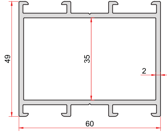
KOD-CODE TEORİK AĞIRLIK 1169 THEORETICAL WEIGHT 1,266 Kg/m
