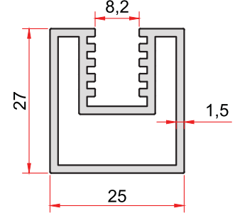
KOD-CODE TEORİK AĞIRLIK 2602 THEORETICAL WEIGHT 0,575 Kg/m
