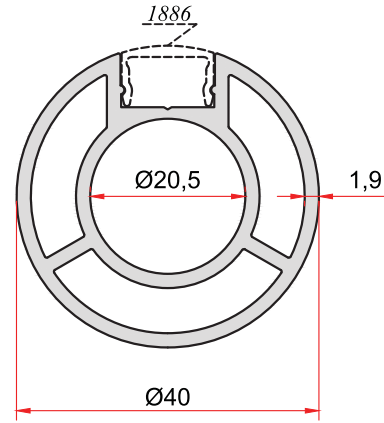
KOD-CODE TEORİK AĞIRLIK 1990 THEORETICAL WEIGHT 1,047 Kg/m
