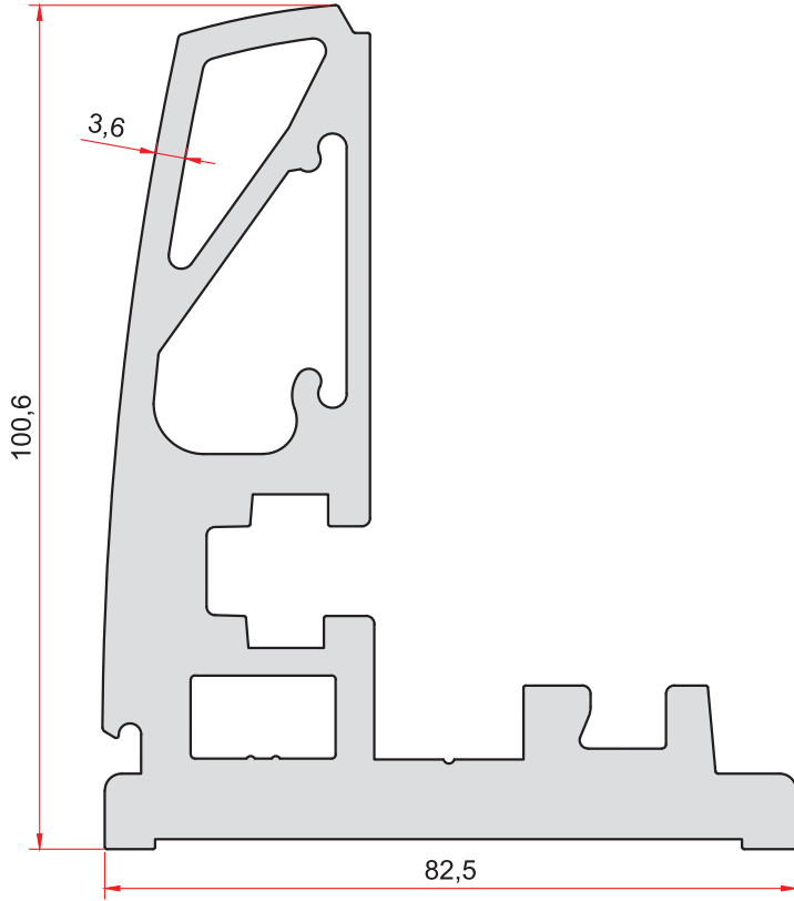
KOD-CODE TEORİK AĞIRLIK THEORETICAL WEIGHT 2277 5,918 Kg/m
