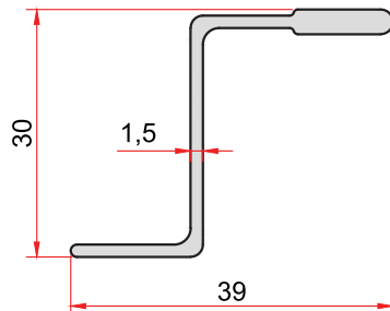
KOD-CODE 1308 TEORİK AĞIRLIK THEORETICAL WEIGHT 0,413 Kg/m
