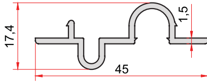
KOD-CODE TEORİK AĞIRLIK 813 0,302 Kg/m
