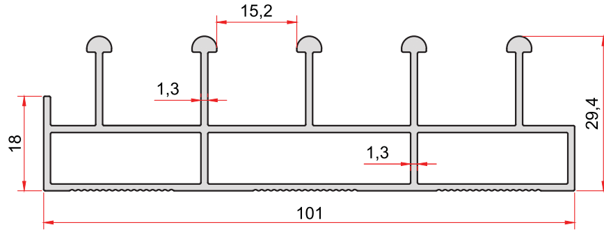
KOD-CODE TEORİK AĞIRLIK THEORETICAL WEIGHT 2439 1,253 Kg/m
