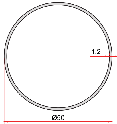
KOD-CODE TEORİK AĞIRLIK 5059 THEORETICAL WEIGHT 0,496 Kg/m
