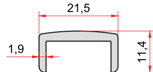
KOD-CODE TEORİK AĞIRLIK 1122 THEORETICAL WEIGHT 0,229 Kg/m
