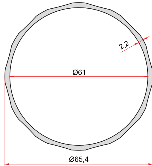
KOD-CODE TEORİK AĞIRLIK THEORETICAL WEIGHT 1887 1,037 Kg/m
