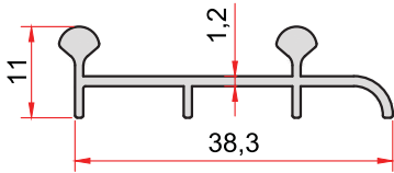
KOD-CODE TEORİK AĞIRLIK THEORETICAL WEIGHT 1402 0,246 Kg/m
