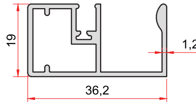
KOD-CODE TEORİK AĞIRLIK THEORETICAL WEIGHT 1427 0,427 Kg/m
