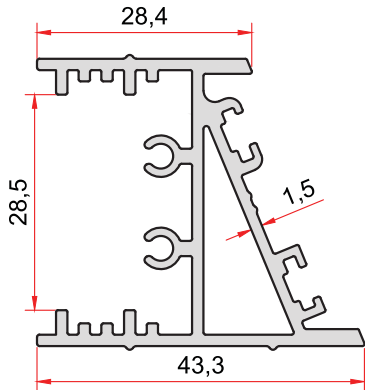
KOD-CODE 2633 TEORİK AĞIRLIK THEORETICAL WEIGHT 0,843 Kg/m
