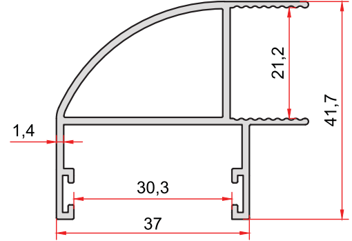
KOD-CODE 2668 TEORİK AĞIRLIK THEORETICAL WEIGHT 0,621 Kg/m
