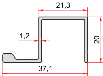
KOD-CODE 1374 TEORİK AĞIRLIK THEORETICAL WEIGHT 0,281 Kg/m
