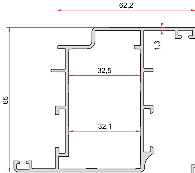
KOD-CODE TEORİK AĞIRLIK THEORETICAL WEIGHT 7036 1,047 Kg/m
