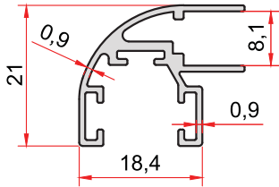
KOD-CODE TEORİK AĞIRLIK 2265 THEORETICAL WEIGHT 0,265 Kg/m
