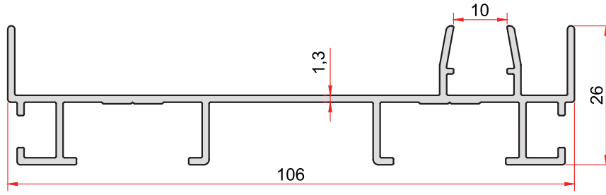
KOD-CODE TEORİK AĞIRLIK THEORETICAL WEIGHT 1024 0,859 Kg/m
