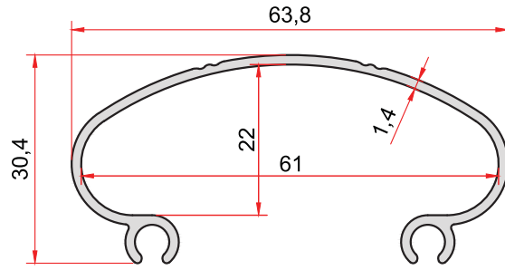
KOD-CODE TEORİK AĞIRLIK 5066 THEORETICAL WEIGHT 0,505 Kg/m
