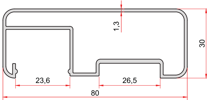
KOD-CODE 5006 TEORİK AĞIRLIK THEORETICAL WEIGHT 0,915 Kg/m
