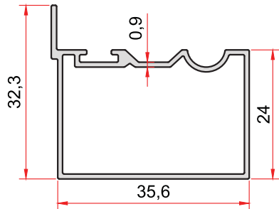
KOD-CODE TEORİK AĞIRLIK 2300 THEORETICAL WEIGHT 0,343 Kg/m
