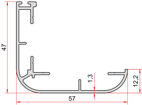
KOD-CODE 1019 TEORİK AĞIRLIK THEORETICAL WEIGHT 0,588 Kg/m
