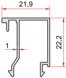
KOD-CODE TEORİK AĞIRLIK THEORETICAL WEIGHT 1131 0,240 Kg/m
