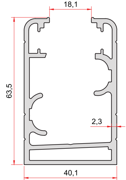
KOD-CODE 2393 TEORİK AĞIRLIK 1,477 Kg/m THEORETICAL WEIGHT
