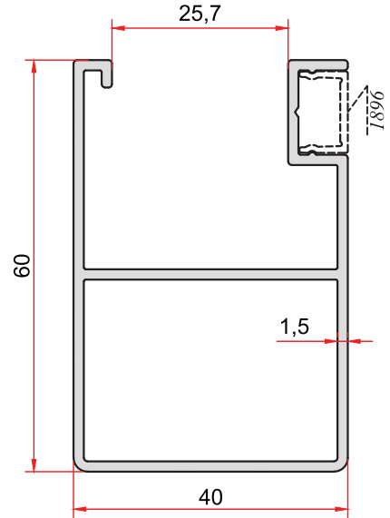
KOD-CODE TEORİK AĞIRLIK 5048 THEORETICAL WEIGHT 0,866 Kg/m
