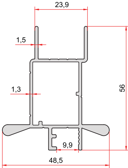
KOD-CODE TEORİK AĞIRLIK 2724 THEORETICAL WEIGHT 0,829 Kg/m
