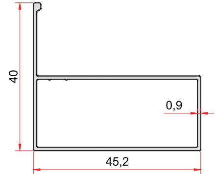
KOD-CODE 771 TEORİK AĞIRLIK THEORETICAL WEIGHT 0,364 Kg/m
