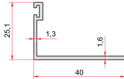
KOD-CODE 7011 TEORİK AĞIRLIK THEORETICAL WEIGHT 0,286 Kg/m
