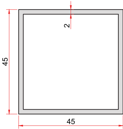
KOD-CODE TEORİK AĞIRLIK THEORETICAL WEIGHT 61 0,929 Kg/m
