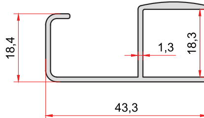
KOD-CODE TEORİK AĞIRLIK THEORETICAL WEIGHT 1507 0,367 Kg/m
