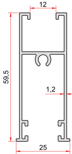
KOD-CODE TEORİK AĞIRLIK 1020 THEORETICAL WEIGHT 0,599 Kg/m
