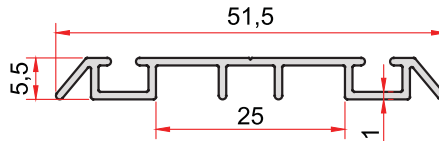
KOD-CODE TEORİK AĞIRLIK THEORETICAL WEIGHT 1359 0,240 Kg/m
