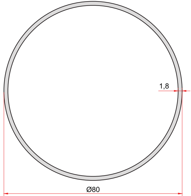
KOD-CODE TEORİK AĞIRLIK THEORETICAL WEIGHT 1936 1,193 Kg/m
