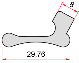
KOD-CODE 1475 TEORİK AĞIRLIK THEORETICAL WEIGHT 0,480 Kg/m
