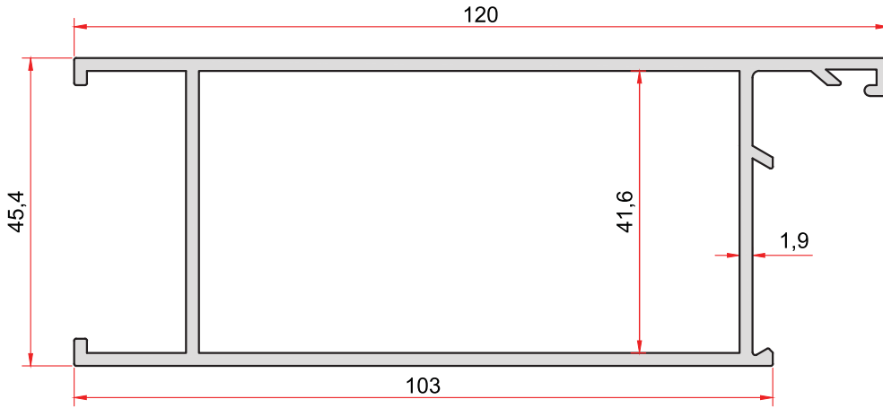
KOD-CODE TEORİK AĞIRLIK THEORETICAL WEIGHT 883 1,642 Kg/m
