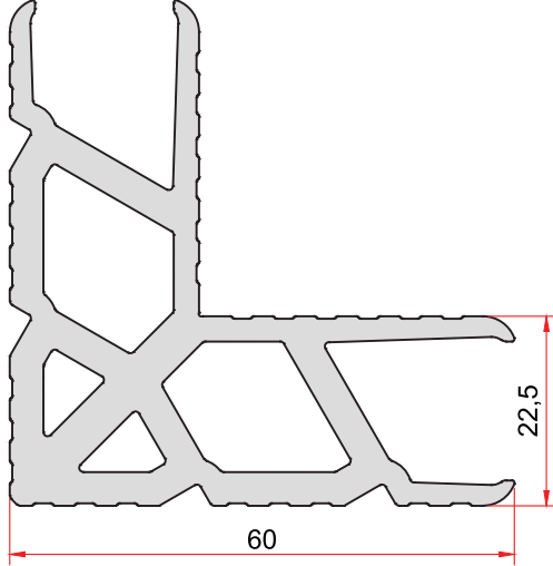
KOD-CODE TEORİK AĞIRLIK THEORETICAL WEIGHT KT-2225-00 2,543 Kg/m
