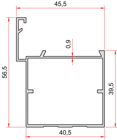
KOD-CODE TEORİK AĞIRLIK 858 THEORETICAL WEIGHT 0,543 Kg/m
