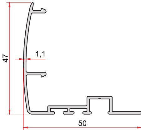
KOD-CODE TEORİK AĞIRLIK SS-602-11 THEORETICAL WEIGHT 0,402 Kg/m
