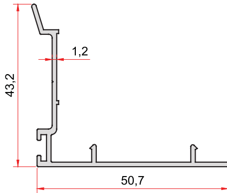
KOD-CODE TEORİK AĞIRLIK 809 THEORETICAL WEIGHT 0,370 Kg/m
