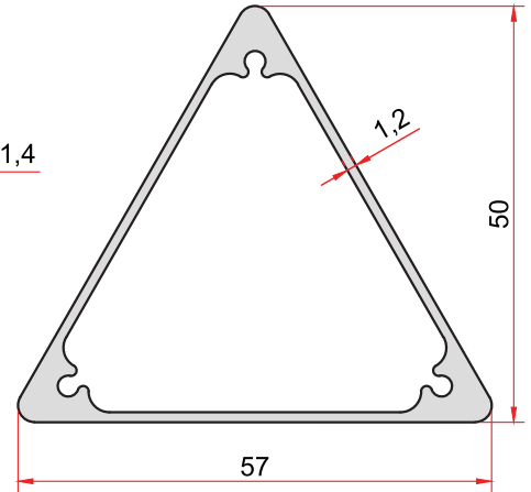
KOD-CODE TEORİK AĞIRLIK THEORETICAL WEIGHT 4018 0,788 Kg/m
