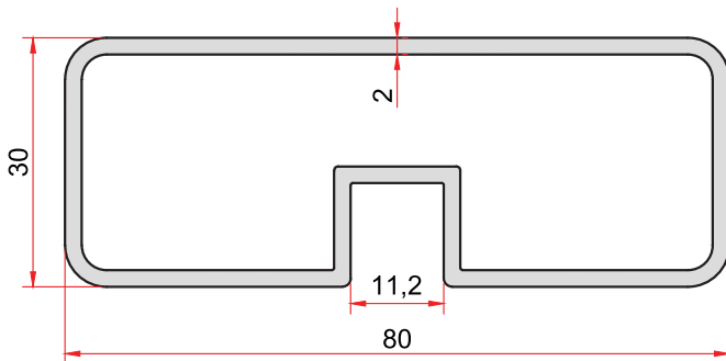
KOD-CODE TEORİK AĞIRLIK 1954 THEORETICAL WEIGHT 1,242 Kg/m
