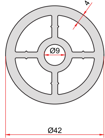
KOD-CODE TEORİK AĞIRLIK 1920 THEORETICAL WEIGHT 1,857 Kg/m
