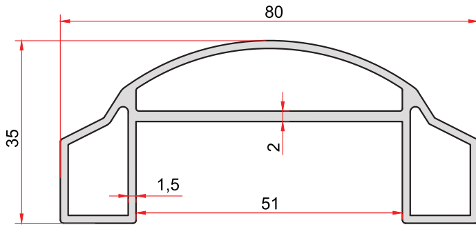
KOD-CODE TEORİK AĞIRLIK 148 THEORETICAL WEIGHT 1,075 Kg/m
