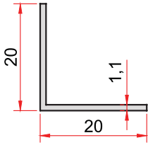
KOD-CODE 14 TEORİK AĞIRLIK THEORETICAL WEIGHT 0,117 Kg/m
