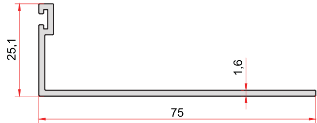
KOD-CODE TEORİK AĞIRLIK THEORETICAL WEIGHT 155 0,454 Kg/m
