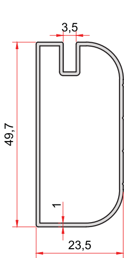
KOD-CODE TEORİK AĞIRLIK THEORETICAL WEIGHT 877 0,402 Kg/m
