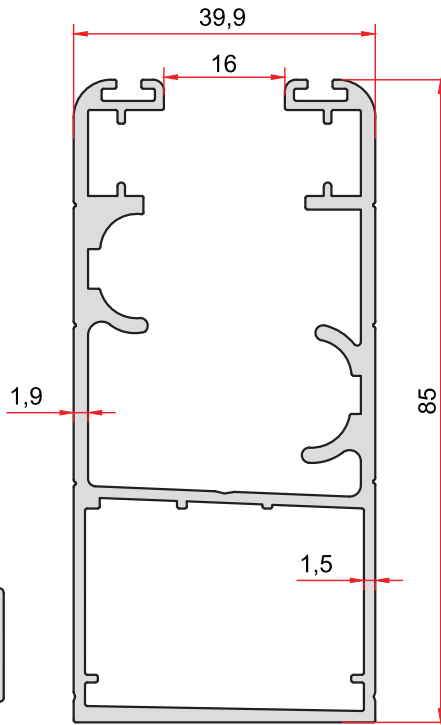
KOD-CODE TEORİK AĞIRLIK THEORETICAL WEIGHT 2373 1,334 Kg/m
