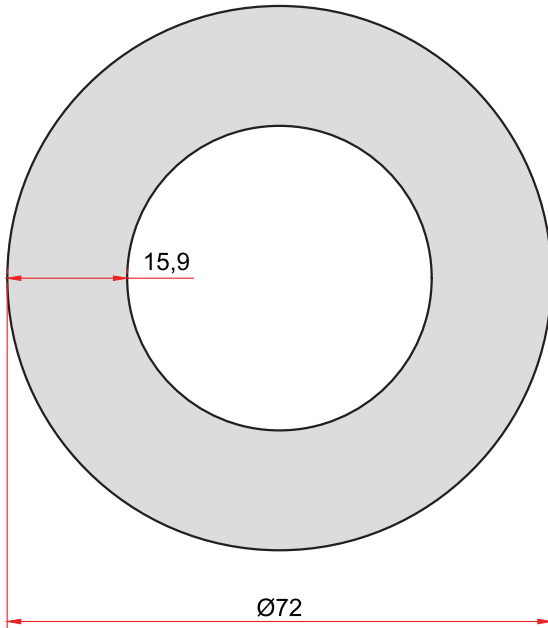
KOD-CODE TEORİK AĞIRLIK THEORETICAL WEIGHT 1852 7,549 Kg/m
