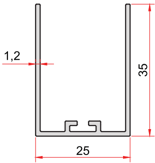
KOD-CODE TEORİK AĞIRLIK THEORETICAL WEIGHT 2437 0,332 Kg/m
