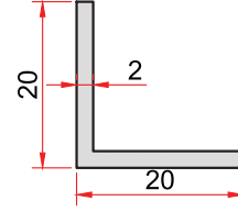
KOD-CODE 34 TEORİK AĞIRLIK THEORETICAL WEIGHT 0,205 Kg/m
