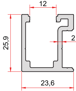
KOD-CODE TEORİK AĞIRLIK 1959 THEORETICAL WEIGHT 0,475 Kg/m
