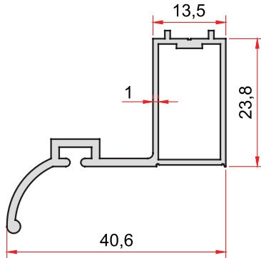
KOD-CODE TEORİK AĞIRLIK THEORETICAL WEIGHT 1780 0,399 Kg/m
