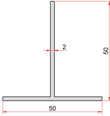
KOD-CODE 78 TEORİK AĞIRLIK THEORETICAL WEIGHT 0,529 Kg/m
