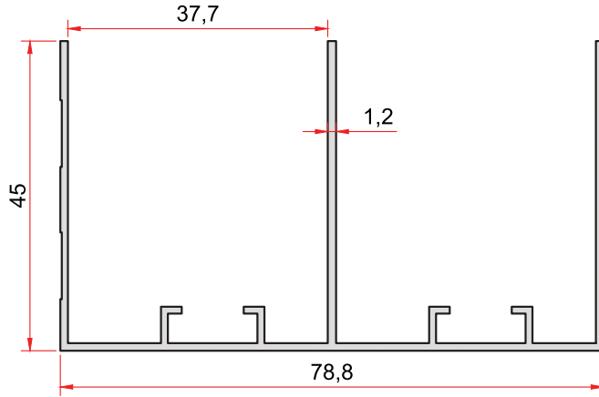
KOD-CODE TEORİK AĞIRLIK THEORETICAL WEIGHT 1482 0,694 Kg/m
