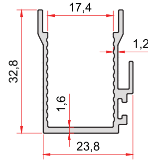
KOD-CODE TEORİK AĞIRLIK THEORETICAL WEIGHT 2387 0,340 Kg/m
