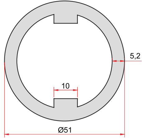
KOD-CODE TEORİK AĞIRLIK THEORETICAL WEIGHT 1861 2,257 Kg/m
