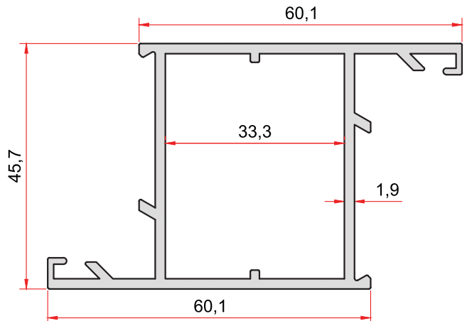
KOD-CODE TEORİK AĞIRLIK 881 THEORETICAL WEIGHT 1,177 Kg/m
