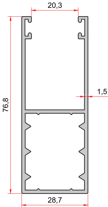
KOD-CODE 1075 TEORİK AĞIRLIK THEORETICAL WEIGHT 0,953 Kg/m
