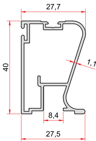
KOD-CODE 1393 TEORİK AĞIRLIK THEORETICAL WEIGHT 0,505 Kg/m
