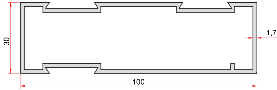
KOD-CODE TEORİK AĞIRLIK 808 THEORETICAL WEIGHT 1,253 Kg/m
