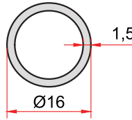
KOD-CODE 1885 TEORİK AĞIRLIK THEORETICAL WEIGHT 0,184 Kg/m
