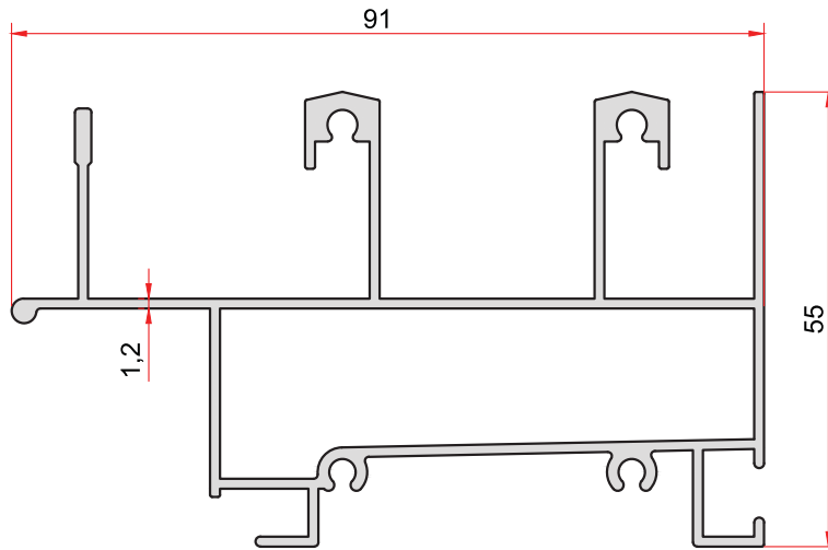
KOD-CODE TEORİK AĞIRLIK THEORETICAL WEIGHT 7004 1,358 Kg/m
