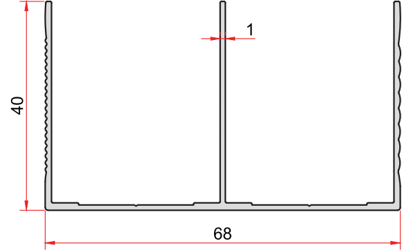
KOD-CODE TEORİK AĞIRLIK THEORETICAL WEIGHT 1458 0,543 Kg/m
