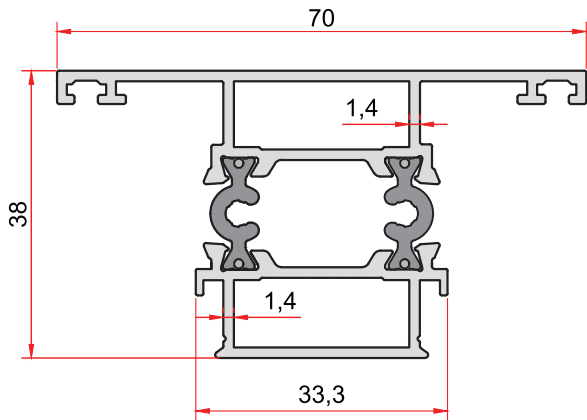
KOD-CODE TEORİK AĞIRLIK İD-301-14 THEORETICAL WEIGHT 1,086 Kg/m
