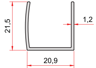
KOD-CODE TEORİK AĞIRLIK THEORETICAL WEIGHT 1379 0,200 Kg/m
