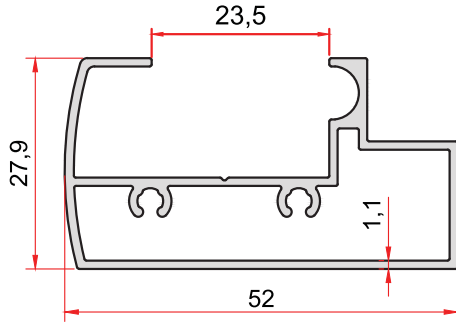
KOD-CODE TEORİK AĞIRLIK 1754 THEORETICAL WEIGHT 0,596 Kg/m
