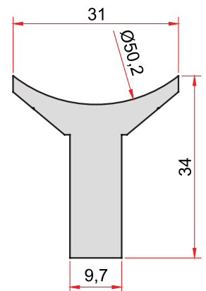
KOD-CODE TEORİK AĞIRLIK THEORETICAL WEIGHT 1862 1,007 Kg/m
