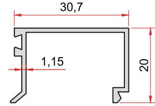
KOD-CODE TEORİK AĞIRLIK 859 THEORETICAL WEIGHT 0,248 Kg/m
