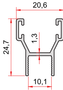
KOD-CODE TEORİK AĞIRLIK 2376 THEORETICAL WEIGHT 0,224 Kg/m
