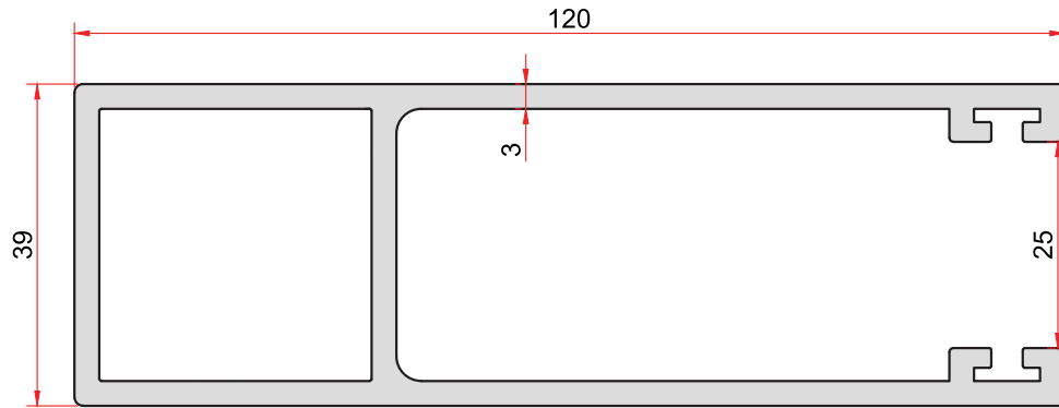
KOD-CODE TEORİK AĞIRLIK THEORETICAL WEIGHT 2312 2,670 Kg/m
