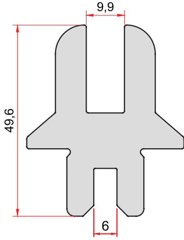
KOD-CODE TEORİK AĞIRLIK THEORETICAL WEIGHT 1856 2,530 Kg/m
