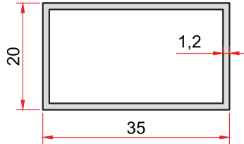
KOD-CODE TEORİK AĞIRLIK 96 THEORETICAL WEIGHT 0,340 Kg/m
