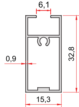
KOD-CODE 1759 TEORİK AĞIRLIK THEORETICAL WEIGHT 0,278 Kg/m
