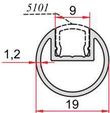
KOD-CODE TEORİK AĞIRLIK 5100 THEORETICAL WEIGHT 0,218 Kg/m
