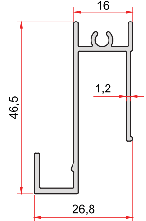
KOD-CODE 1469 TEORİK AĞIRLIK THEORETICAL WEIGHT 0,413 Kg/m
