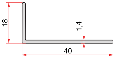
KOD-CODE 156 TEORİK AĞIRLIK THEORETICAL WEIGHT 0,211 Kg/m
