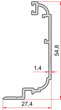
KOD-CODE TEORİK AĞIRLIK İS-402-14 THEORETICAL WEIGHT 0,375 Kg/m
