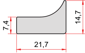
KOD-CODE 1497 TEORİK AĞIRLIK THEORETICAL WEIGHT 0,505 Kg/m
