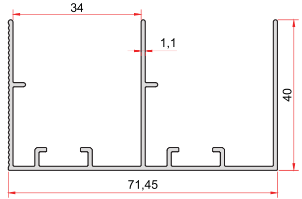
KOD-CODE TEORİK AĞIRLIK THEORETICAL WEIGHT 1485 0,661 Kg/m
