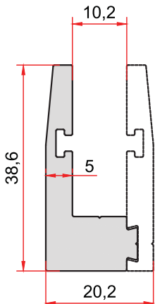
KOD-CODE 5098 TEORİK AĞIRLIK THEORETICAL WEIGHT 0,769 Kg/m
