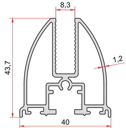
KOD-CODE TEORİK AĞIRLIK THEORETICAL WEIGHT 2637 0,847 Kg/m
