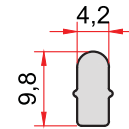
KOD-CODE TEORİK AĞIRLIK THEORETICAL WEIGHT SS-507-00 0,108 Kg/m
