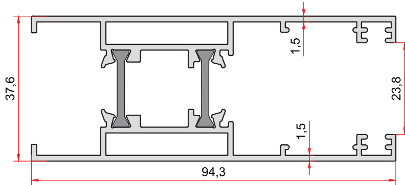
KOD-CODE TEORİK AĞIRLIK THEORETICAL WEIGHT MD-101-15 1,616 Kg/m
