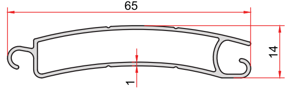
KOD-CODE TEORİK AĞIRLIK 2316 THEORETICAL WEIGHT 0,410 Kg/m
