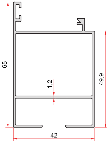
KOD-CODE TEORİK AĞIRLIK THEORETICAL WEIGHT 782 0,788 Kg/m
