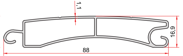
KOD-CODE TEORİK AĞIRLIK 2315 THEORETICAL WEIGHT 0,667 Kg/m
