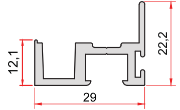
KOD-CODE 1367 TEORİK AĞIRLIK THEORETICAL WEIGHT 0,408 Kg/m
