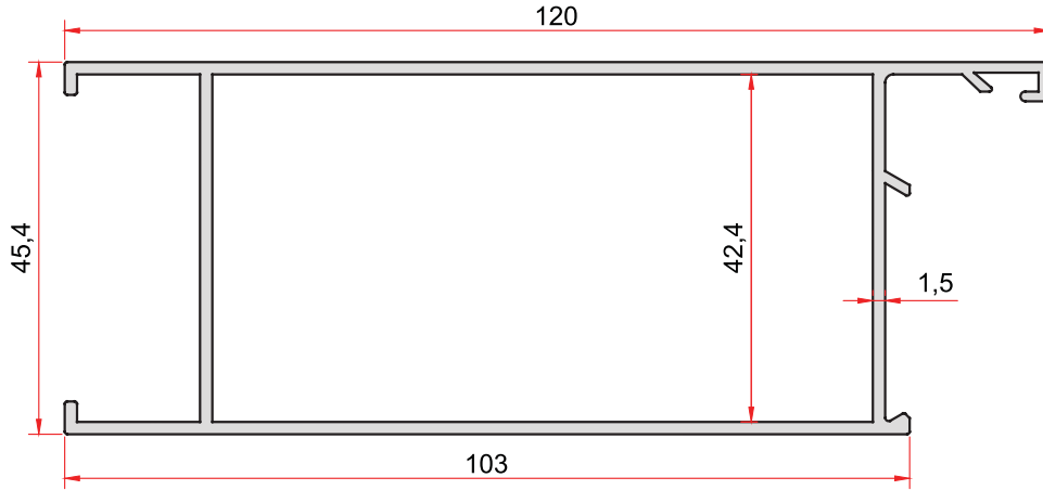
KOD-CODE TEORİK AĞIRLIK THEORETICAL WEIGHT 831 1,307 Kg/m
