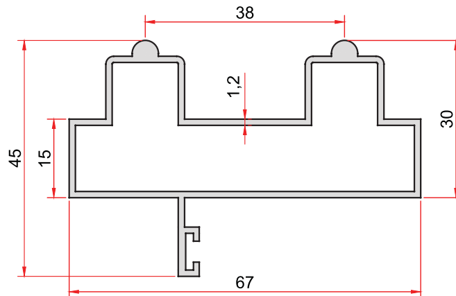
KOD-CODE TEORİK AĞIRLIK THEORETICAL WEIGHT 816 0,810 Kg/m
