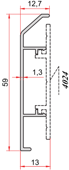
KOD-CODE 4025 TEORİK AĞIRLIK THEORETICAL WEIGHT 0,305 Kg/m
