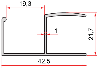
KOD-CODE TEORİK AĞIRLIK THEORETICAL WEIGHT 1387 0,294 Kg/m
