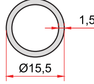
KOD-CODE 1922 TEORİK AĞIRLIK THEORETICAL WEIGHT 0,178 Kg/m
