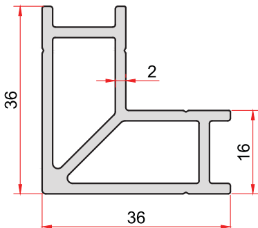
KOD-CODE TEORİK AĞIRLIK 1160 THEORETICAL WEIGHT 0,831 Kg/m
