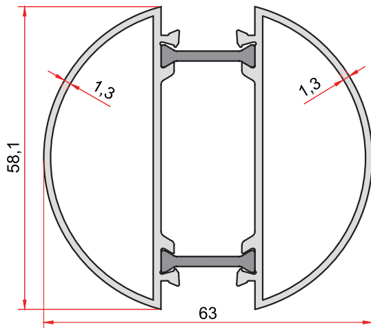
KOD-CODE TEORİK AĞIRLIK İD-901-13 THEORETICAL WEIGHT 1,251 Kg/m
