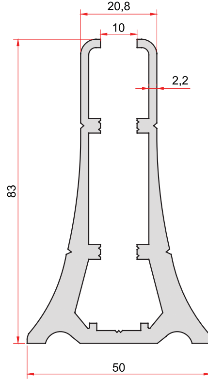
KOD-CODE TEORİK AĞIRLIK THEORETICAL WEIGHT 1877 2,349 Kg/m
