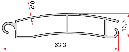
KOD-CODE TEORİK AĞIRLIK 2313 THEORETICAL WEIGHT 0,402 Kg/m
