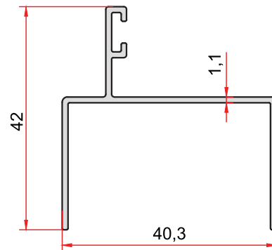
KOD-CODE 2667 TEORİK AĞIRLIK THEORETICAL WEIGHT 0,337 Kg/m
