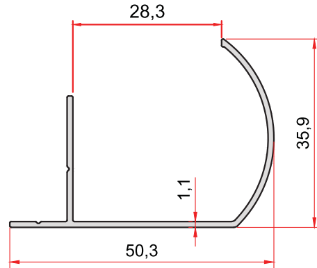
KOD-CODE 1756 TEORİK AĞIRLIK THEORETICAL WEIGHT 0,313 Kg/m
