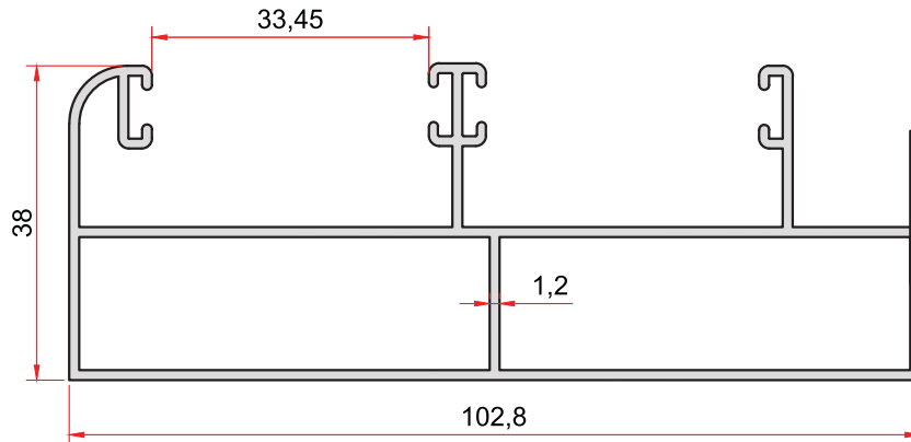
KOD-CODE TEORİK AĞIRLIK 872 THEORETICAL WEIGHT 1,215 Kg/m
