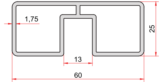
KOD-CODE TEORİK AĞIRLIK 1997 THEORETICAL WEIGHT 0,937 Kg/m
