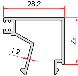
KOD-CODE TEORİK AĞIRLIK THEORETICAL WEIGHT 1145 0,324 Kg/m
