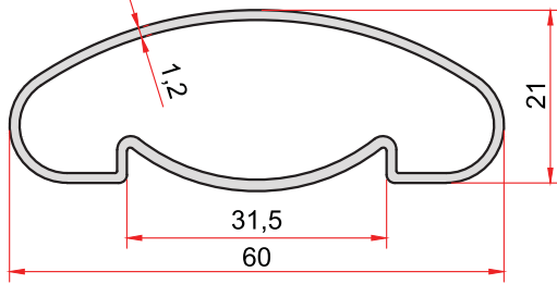
KOD-CODE 5033 TEORİK AĞIRLIK THEORETICAL WEIGHT 0,489 Kg/m
