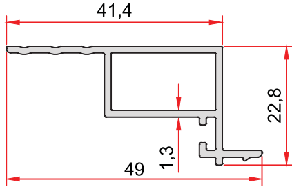
KOD-CODE TEORİK AĞIRLIK THEORETICAL WEIGHT AO-1021-13 0,384 Kg/m
