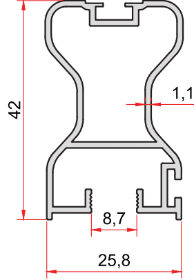
KOD-CODE 1365 TEORİK AĞIRLIK THEORETICAL WEIGHT 0,516 Kg/m
