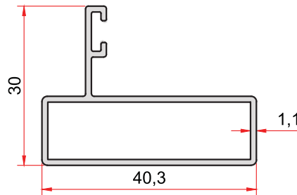
KOD-CODE TEORİK AĞIRLIK 2256 THEORETICAL WEIGHT 0,378 Kg/m
