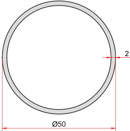
KOD-CODE TEORİK AĞIRLIK THEORETICAL WEIGHT 1881 0,815 Kg/m
