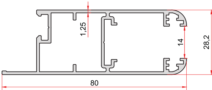
KOD-CODE TEORİK AĞIRLIK 7026 THEORETICAL WEIGHT 0,880 Kg/m
