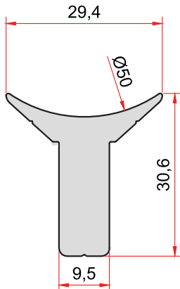
KOD-CODE TEORİK AĞIRLIK THEORETICAL WEIGHT 1942 0,853 Kg/m
