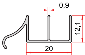
KOD-CODE 777 TEORİK AĞIRLIK THEORETICAL WEIGHT 0,176 Kg/m
