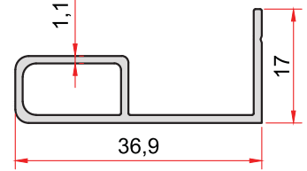
KOD-CODE TEORİK AĞIRLIK THEORETICAL WEIGHT 1430 0,267 Kg/m
