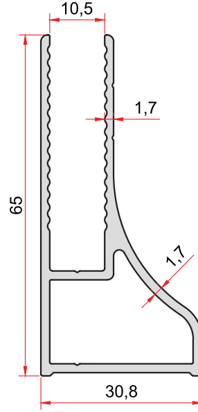
KOD-CODE TEORİK AĞIRLIK 1914 THEORETICAL WEIGHT 0,826 Kg/m
