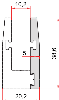
KOD-CODE 5099 TEORİK AĞIRLIK THEORETICAL WEIGHT 0,421 Kg/m
