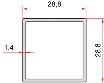
KOD-CODE TEORİK AĞIRLIK 5083 THEORETICAL WEIGHT 0,413 Kg/m
