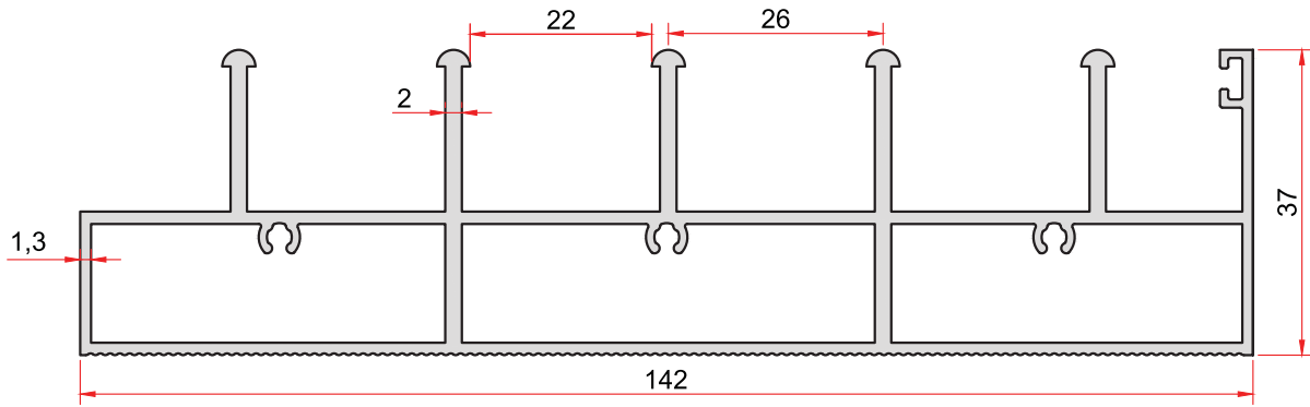
KOD-CODE TEORİK AĞIRLIK THEORETICAL WEIGHT 2382 2,084 Kg/m
