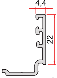
KOD-CODE TEORİK AĞIRLIK CC-1044-15 THEORETICAL WEIGHT 0,212 Kg/m
