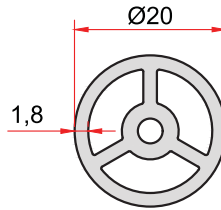
KOD-CODE TEORİK AĞIRLIK THEORETICAL WEIGHT 1496 0,440 Kg/m
