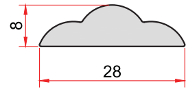
KOD-CODE TEORİK AĞIRLIK THEORETICAL WEIGHT 1444 0,389 Kg/m
