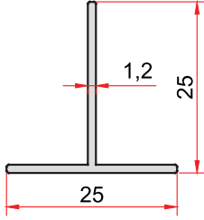
KOD-CODE 19 TEORİK AĞIRLIK THEORETICAL WEIGHT 0,157 Kg/m
