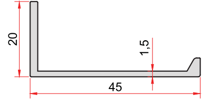
KOD-CODE TEORİK AĞIRLIK THEORETICAL WEIGHT 1487 0,308 Kg/m
