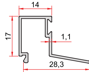
KOD-CODE TEORİK AĞIRLIK THEORETICAL WEIGHT 835 0,205 Kg/m
