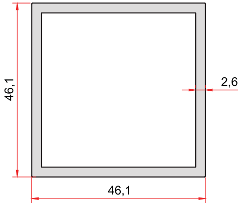
KOD-CODE TEORİK AĞIRLIK 1965 THEORETICAL WEIGHT 1,220 Kg/m
