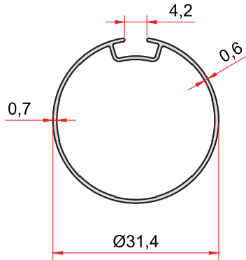
KOD-CODE 2201 TEORİK AĞIRLIK THEORETICAL WEIGHT 0,203 Kg/m
