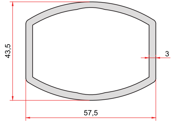
KOD-CODE TEORİK AĞIRLIK 5038 THEORETICAL WEIGHT 1,306 Kg/m
