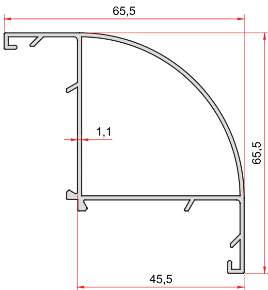
KOD-CODE TEORİK AĞIRLIK THEORETICAL WEIGHT 838 0,699 Kg/m
