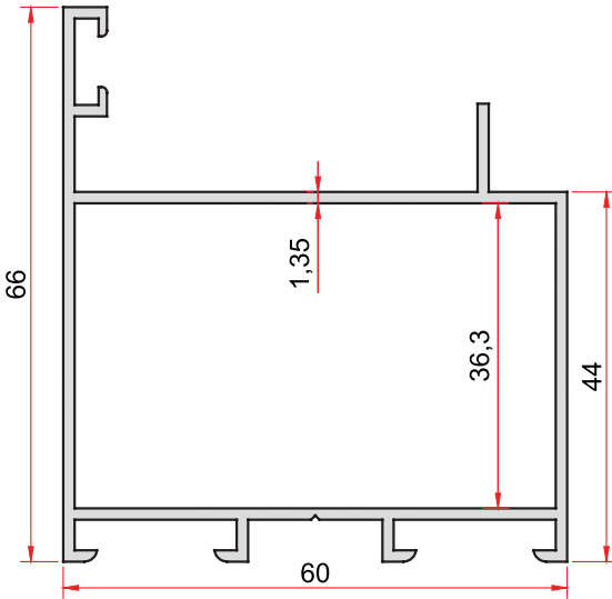
KOD-CODE TEORİK AĞIRLIK 845 THEORETICAL WEIGHT 0,967 Kg/m
