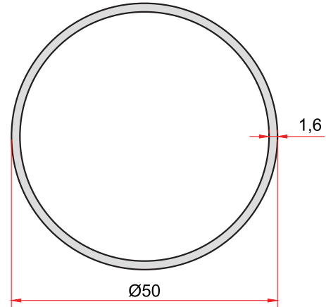
KOD-CODE TEORİK AĞIRLIK THEORETICAL WEIGHT 1912 0,656 Kg/m
