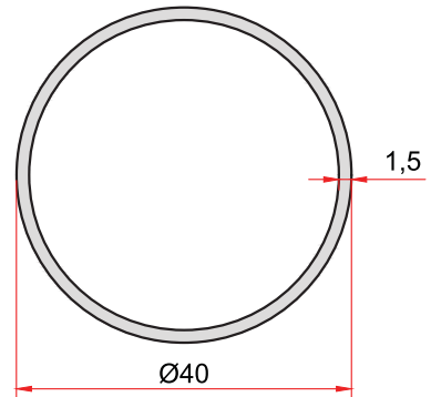
KOD-CODE TEORİK AĞIRLIK 1910 THEORETICAL WEIGHT 0,489 Kg/m
