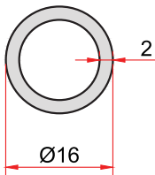
KOD-CODE 1943 TEORİK AĞIRLIK THEORETICAL WEIGHT 0,238 Kg/m
