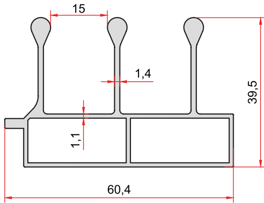
KOD-CODE TEORİK AĞIRLIK 2698 THEORETICAL WEIGHT 0,910 Kg/m
