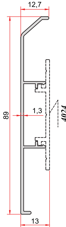
KOD-CODE 4026 TEORİK AĞIRLIK THEORETICAL WEIGHT 0,410 Kg/m
