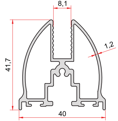
KOD-CODE TEORİK AĞIRLIK THEORETICAL WEIGHT 2261 0,805 Kg/m
