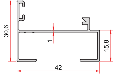
KOD-CODE TEORİK AĞIRLIK THEORETICAL WEIGHT 781 0,348 Kg/m
