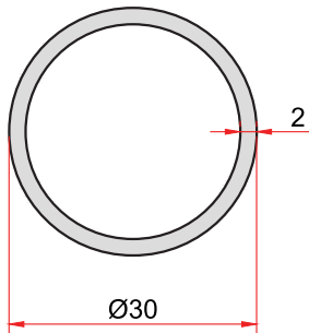
KOD-CODE TEORİK AĞIRLIK 1993 THEORETICAL WEIGHT 0,475 Kg/m
