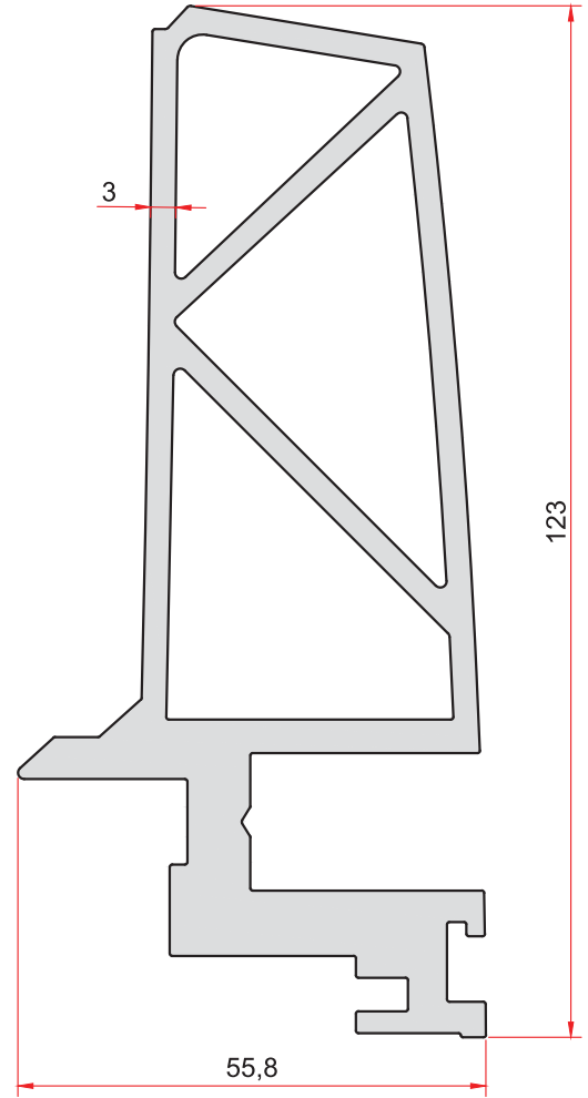
KOD-CODE TEORİK AĞIRLIK 1994 THEORETICAL WEIGHT 4,282 Kg/m
