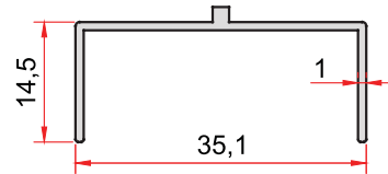
KOD-CODE 795 TEORİK AĞIRLIK THEORETICAL WEIGHT 0,178 Kg/m
