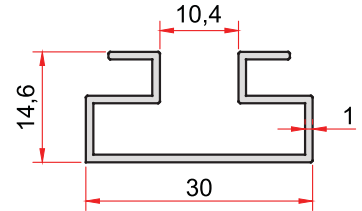
KOD-CODE TEORİK AĞIRLIK THEORETICAL WEIGHT 1389 0,232 Kg/m
