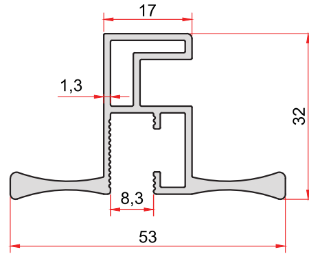
KOD-CODE TEORİK AĞIRLIK THEORETICAL WEIGHT 2446 0,653 Kg/m
