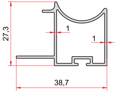
KOD-CODE 1510 TEORİK AĞIRLIK 0,345 Kg/m THEORETICAL WEIGHT
