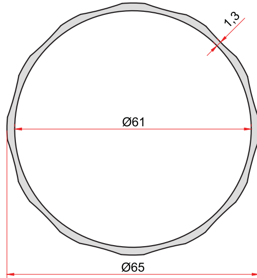
KOD-CODE TEORİK AĞIRLIK THEORETICAL WEIGHT 1917 0,902 Kg/m
