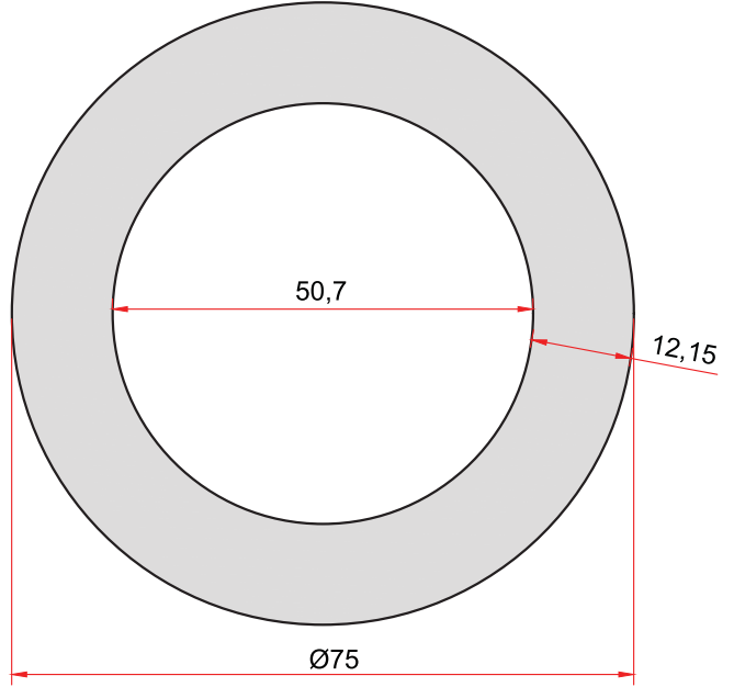
KOD-CODE TEORİK AĞIRLIK THEORETICAL WEIGHT 5068 6,480 Kg/m
