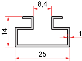
KOD-CODE TEORİK AĞIRLIK THEORETICAL WEIGHT 1391 0,197 Kg/m
