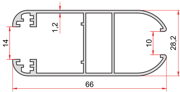
KOD-CODE TEORİK AĞIRLIK THEORETICAL WEIGHT 785 0,726 Kg/m
