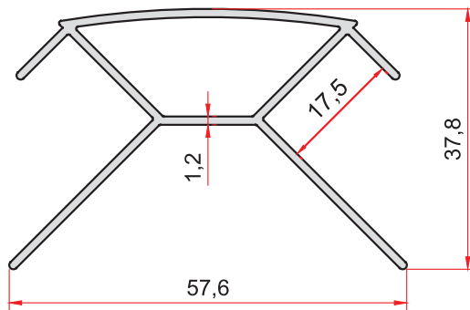
KOD-CODE TEORİK AĞIRLIK THEORETICAL WEIGHT 1785 0,562 Kg/m
