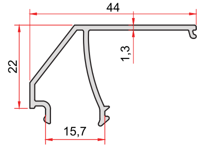
KOD-CODE TEORİK AĞIRLIK 1981 THEORETICAL WEIGHT 0,335 Kg/m
