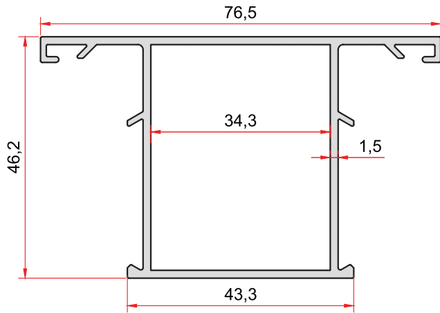
KOD-CODE TEORİK AĞIRLIK 907 THEORETICAL WEIGHT 0,921 Kg/m
