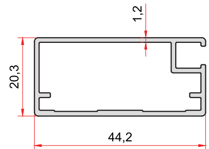
KOD-CODE 1462 TEORİK AĞIRLIK 0,467 Kg/m THEORETICAL WEIGHT
