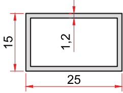
KOD-CODE TEORİK AĞIRLIK 46 THEORETICAL WEIGHT 0,243 Kg/m
