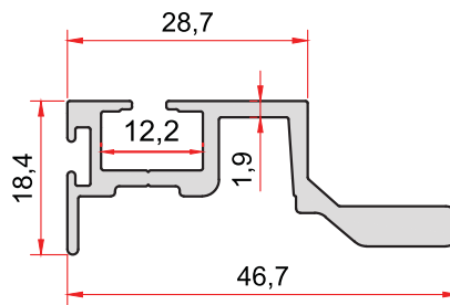
KOD-CODE 1467 TEORİK AĞIRLIK THEORETICAL WEIGHT 0,581 Kg/m
