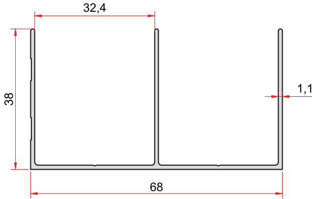
KOD-CODE TEORİK AĞIRLIK THEORETICAL WEIGHT 1371 0,524 Kg/m
