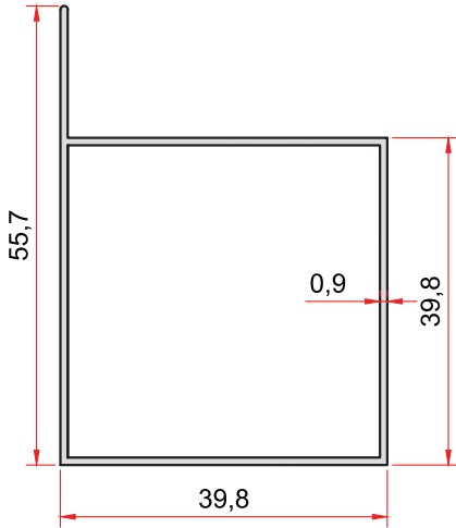
KOD-CODE 1435 TEORİK AĞIRLIK THEORETICAL WEIGHT 0,416 Kg/m
