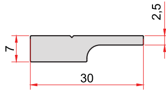
KOD-CODE 1476 TEORİK AĞIRLIK THEORETICAL WEIGHT 0,392 Kg/m
