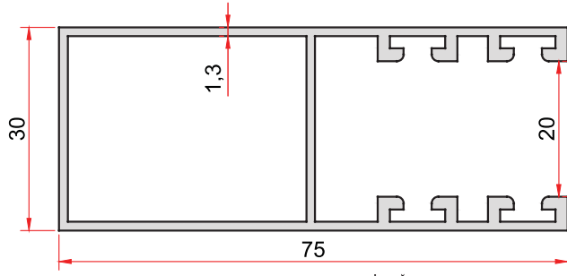
KOD-CODE TEORİK AĞIRLIK THEORETICAL WEIGHT 2306 0,937 Kg/m
