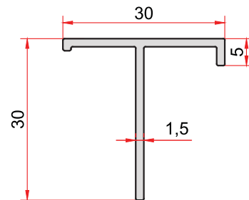
KOD-CODE TEORİK AĞIRLIK 1060 THEORETICAL WEIGHT 0,254 Kg/m
