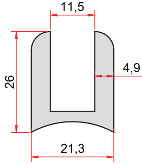
KOD-CODE 1872 TEORİK AĞIRLIK THEORETICAL WEIGHT 0,721 Kg/m
