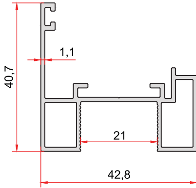
KOD-CODE 2732 TEORİK AĞIRLIK 0,529 Kg/m THEORETICAL WEIGHT
