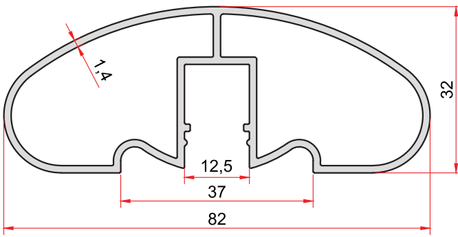
KOD-CODE TEORİK AĞIRLIK THEORETICAL WEIGHT 1998 0,939 Kg/m
