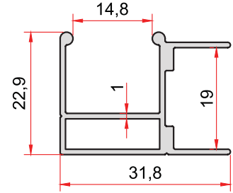
KOD-CODE 1505 TEORİK AĞIRLIK 0,335 Kg/m THEORETICAL WEIGHT
