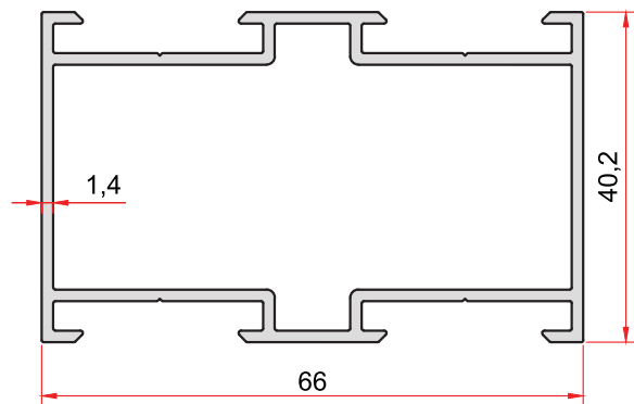
KOD-CODE TEORİK AĞIRLIK 1036 THEORETICAL WEIGHT 0,944 Kg/m
