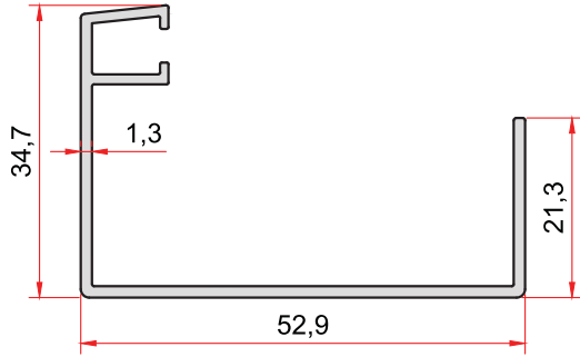
KOD-CODE TEORİK AĞIRLIK 2252 THEORETICAL WEIGHT 0,451 Kg/m
