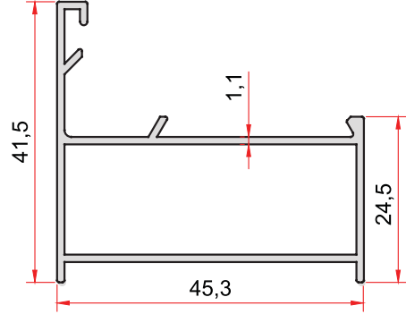
KOD-CODE TEORİK AĞIRLIK 823 THEORETICAL WEIGHT 0,499 Kg/m
