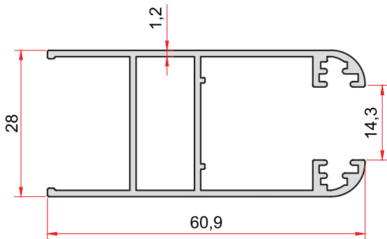
KOD-CODE TEORİK AĞIRLIK THEORETICAL WEIGHT 1067 0,680 Kg/m
