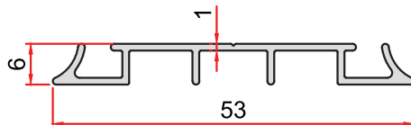
KOD-CODE TEORİK AĞIRLIK THEORETICAL WEIGHT 1456 0,230 Kg/m
