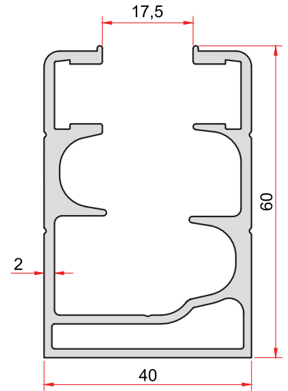
KOD-CODE 2293 TEORİK AĞIRLIK THEORETICAL WEIGHT 1,393 Kg/m
