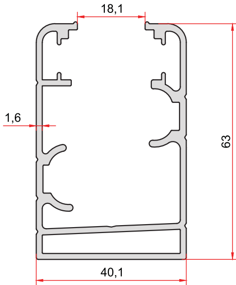
KOD-CODE 2680 TEORİK AĞIRLIK THEORETICAL WEIGHT 1,231 Kg/m
