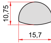
KOD-CODE TEORİK AĞIRLIK THEORETICAL WEIGHT 1491 0,362 Kg/m
