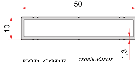
KOD-CODE TEORİK AĞIRLIK 5088 THEORETICAL WEIGHT 0,400 Kg/m
