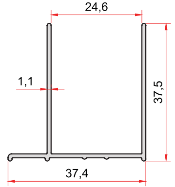
KOD-CODE 1774 TEORİK AĞIRLIK THEORETICAL WEIGHT 0,321 Kg/m
