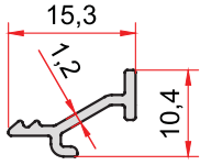
KOD-CODE TEORİK AĞIRLIK THEORETICAL WEIGHT AO-1031-12 0,084 Kg/m
