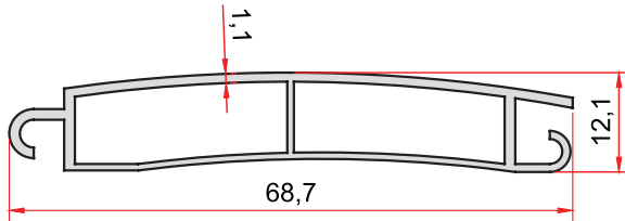
KOD-CODE TEORİK AĞIRLIK 2304 THEORETICAL WEIGHT 0,454 Kg/m
