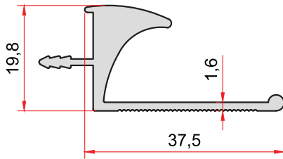
KOD-CODE 1383 TEORİK AĞIRLIK THEORETICAL WEIGHT 0,500 Kg/m
