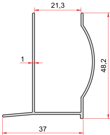
KOD-CODE 1771 TEORİK AĞIRLIK THEORETICAL WEIGHT 0,356 Kg/m
