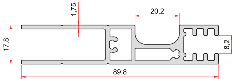
KOD-CODE TEORİK AĞIRLIK THEORETICAL WEIGHT 2444 1,226 Kg/m
