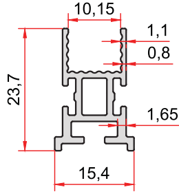
KOD-CODE TEORİK AĞIRLIK 2722 THEORETICAL WEIGHT 0,267 Kg/m
