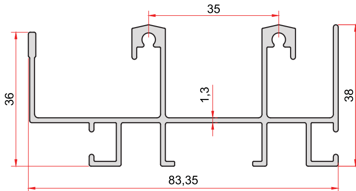
KOD-CODE TEORİK AĞIRLIK THEORETICAL WEIGHT 1079 1,288 Kg/m
