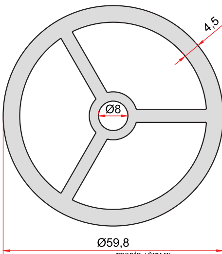
KOD-CODE TEORİK AĞIRLIK 1870 THEORETICAL WEIGHT 2,870 Kg/m
