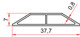
KOD-CODE TEORİK AĞIRLIK THEORETICAL WEIGHT 4002 0,189 Kg/m
