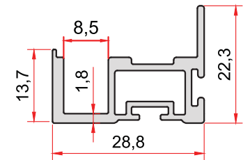
KOD-CODE 1470 TEORİK AĞIRLIK THEORETICAL WEIGHT 0,397 Kg/m
