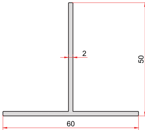
KOD-CODE 81 TEORİK AĞIRLIK THEORETICAL WEIGHT 0,583 Kg/m
