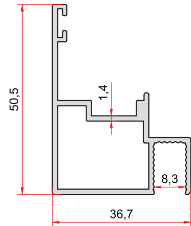
KOD-CODE 2681 TEORİK AĞIRLIK 0,610 Kg/m THEORETICAL WEIGHT
