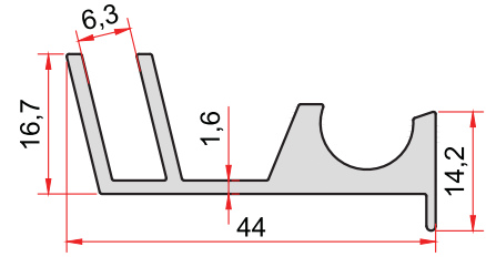
KOD-CODE 105 TEORİK AĞIRLIK THEORETICAL WEIGHT 0,578 Kg/m
