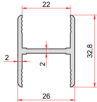
KOD-CODE TEORİK AĞIRLIK 5009 THEORETICAL WEIGHT 0,459 Kg/m
