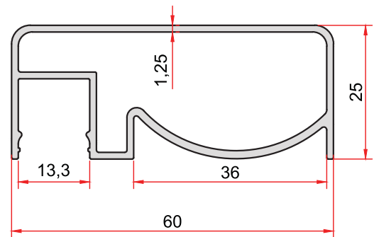
KOD-CODE TEORİK AĞIRLIK THEORETICAL WEIGHT 1961 0,675 Kg/m
