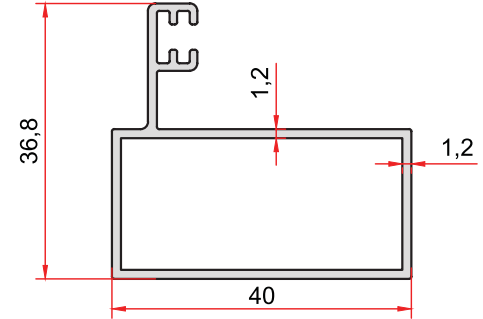
KOD-CODE TEORİK AĞIRLIK 2726 THEORETICAL WEIGHT 0,472 Kg/m
