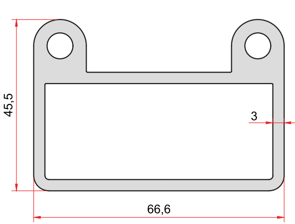
KOD-CODE TEORİK AĞIRLIK 1983 THEORETICAL WEIGHT 2,217 Kg/m
