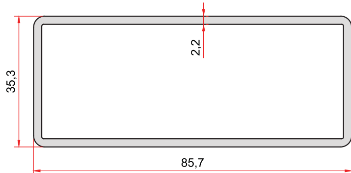
KOD-CODE TEORİK AĞIRLIK 1977 THEORETICAL WEIGHT 1,364 Kg/m
