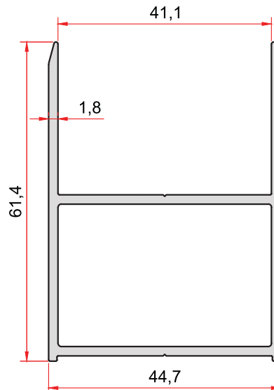
KOD-CODE 2253 TEORİK AĞIRLIK THEORETICAL WEIGHT 0,983 Kg/m
