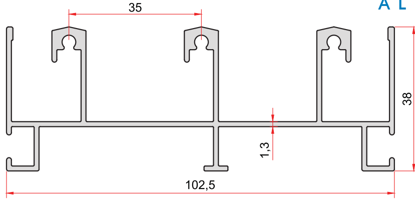
KOD-CODE TEORİK AĞIRLIK THEORETICAL WEIGHT 1009 1,307 Kg/m
