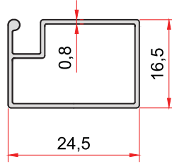
KOD-CODE 1302 TEORİK AĞIRLIK THEORETICAL WEIGHT 0,191 Kg/m
