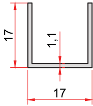
KOD-CODE TEORİK AĞIRLIK 83 THEORETICAL WEIGHT 0,146 Kg/m
