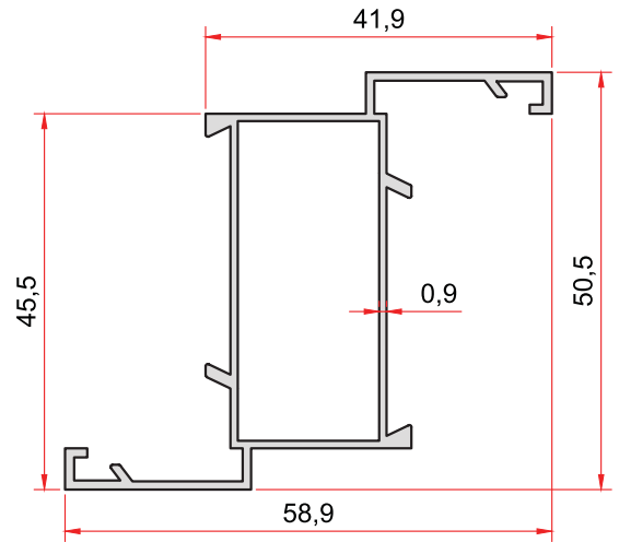
KOD-CODE TEORİK AĞIRLIK 861 THEORETICAL WEIGHT 0,537 Kg/m
