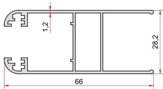
KOD-CODE TEORİK AĞIRLIK THEORETICAL WEIGHT 851 0,699 Kg/m
