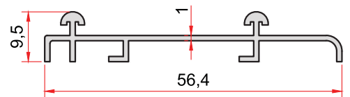
KOD-CODE TEORİK AĞIRLIK THEORETICAL WEIGHT 1376 0,275 Kg/m
