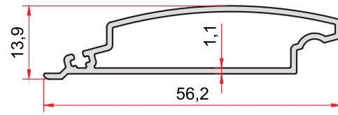
KOD-CODE 1015 TEORİK AĞIRLIK THEORETICAL WEIGHT 0,365 Kg/m
