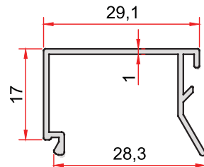
KOD-CODE TEORİK AĞIRLIK THEORETICAL WEIGHT 833 0,208 Kg/m
