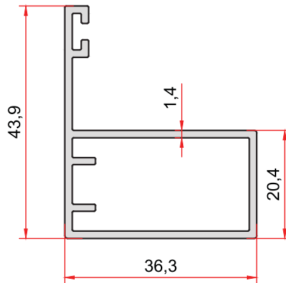
KOD-CODE 2756 TEORİK AĞIRLIK THEORETICAL WEIGHT 0,564 Kg/m
