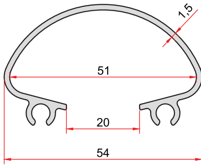
KOD-CODE TEORİK AĞIRLIK 5051 THEORETICAL WEIGHT 0,548 Kg/m
