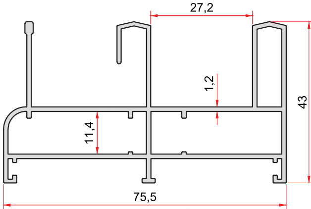
KOD-CODE TEORİK AĞIRLIK THEORETICAL WEIGHT 1065 1,069 Kg/m
