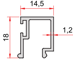
KOD-CODE TEORİK AĞIRLIK 817 THEORETICAL WEIGHT 0,194 Kg/m
