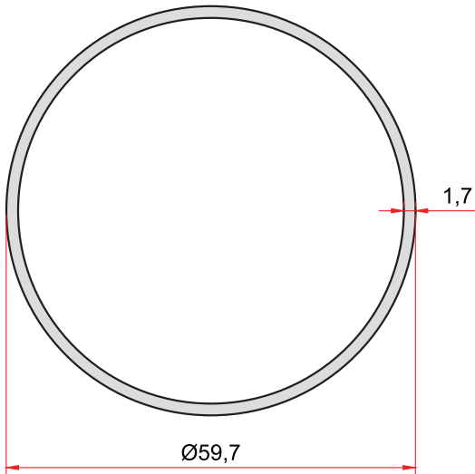
KOD-CODE TEORİK AĞIRLIK THEORETICAL WEIGHT 1902 0,837 Kg/m
