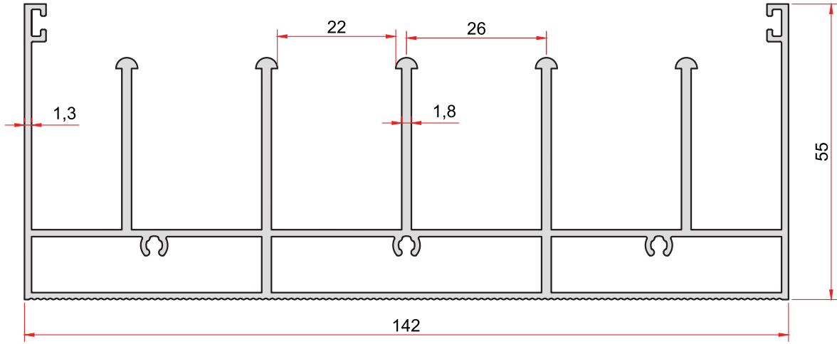
KOD-CODE TEORİK AĞIRLIK THEORETICAL WEIGHT 2381 2,349 Kg/m
