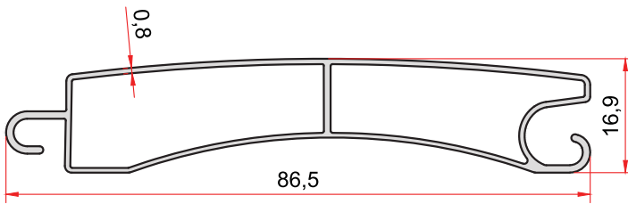
KOD-CODE TEORİK AĞIRLIK 2310 THEORETICAL WEIGHT 0,486 Kg/m
