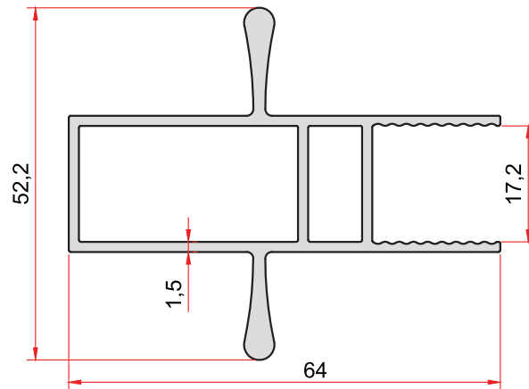
KOD-CODE TEORİK AĞIRLIK THEORETICAL WEIGHT 2385 0,956 Kg/m
