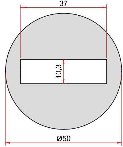
KOD-CODE 1863 TEORİK AĞIRLIK THEORETICAL WEIGHT 4,271 Kg/m
