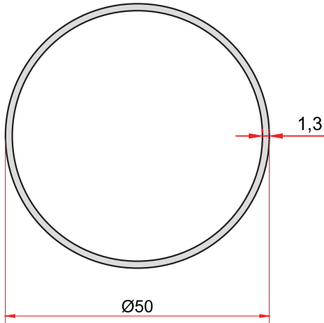
KOD-CODE TEORİK AĞIRLIK THEORETICAL WEIGHT 1957 0,537 Kg/m
