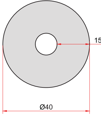
KOD-CODE 1853 TEORİK AĞIRLIK THEORETICAL WEIGHT 3,181 Kg/m
