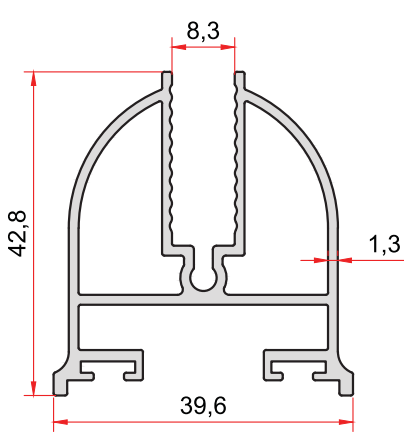
KOD-CODE TEORİK AĞIRLIK THEORETICAL WEIGHT 2251 0,775 Kg/m
