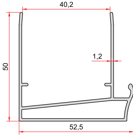
KOD-CODE 2664 TEORİK AĞIRLIK THEORETICAL WEIGHT 0,680 Kg/m
