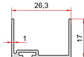
KOD-CODE TEORİK AĞIRLIK 2758 THEORETICAL WEIGHT 0,180 Kg/m
