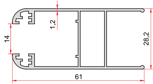
KOD-CODE TEORİK AĞIRLIK THEORETICAL WEIGHT 786 0,667 Kg/m
