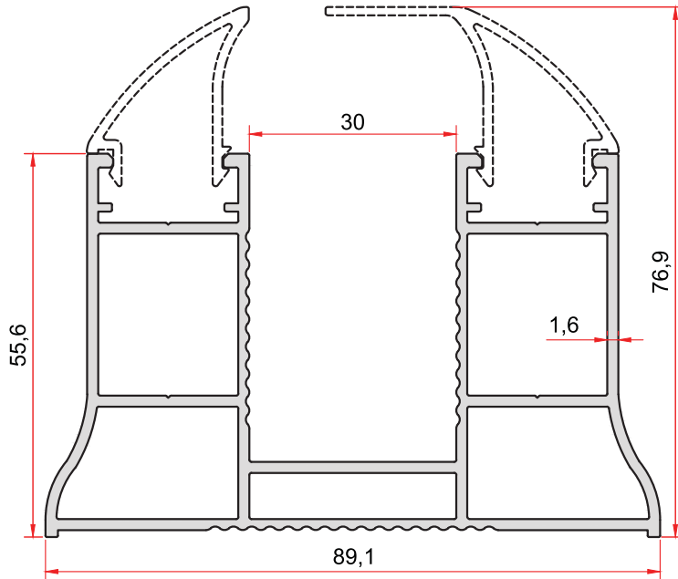
KOD-CODE TEORİK AĞIRLIK 5017 THEORETICAL WEIGHT 1,804 Kg/m
