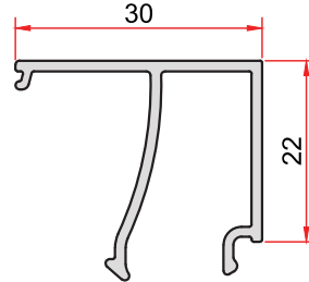
KOD-CODE TEORİK AĞIRLIK CC-1300-13 THEORETICAL WEIGHT 0,305 Kg/m
