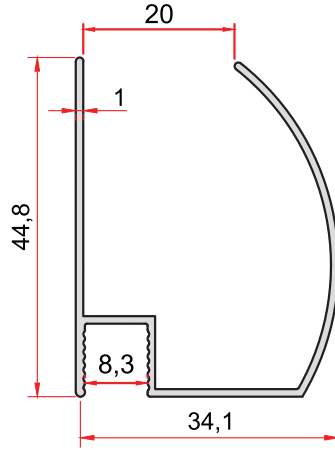
KOD-CODE TEORİK AĞIRLIK THEORETICAL WEIGHT 1764 0,353 Kg/m
