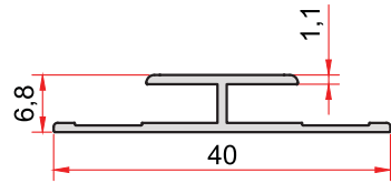
KOD-CODE TEORİK AĞIRLIK 1061 THEORETICAL WEIGHT 0,173 Kg/m
