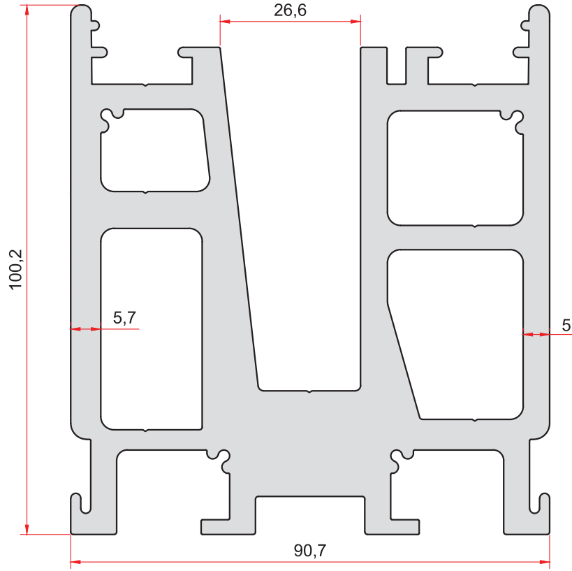
KOD-CODE TEORİK AĞIRLIK 1945 THEORETICAL WEIGHT 9,310 Kg/m
