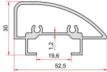
KOD-CODE TEORİK AĞIRLIK 1775 THEORETICAL WEIGHT 0,726 Kg/m
