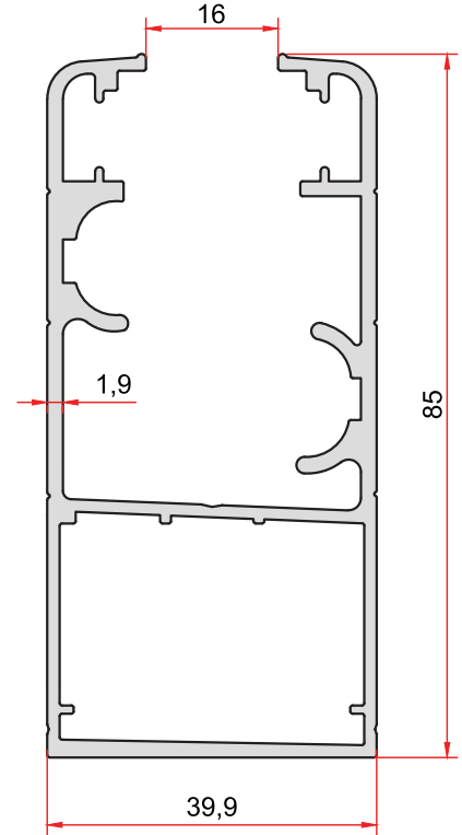
KOD-CODE TEORİK AĞIRLIK 2730 THEORETICAL WEIGHT 1,547 Kg/m
