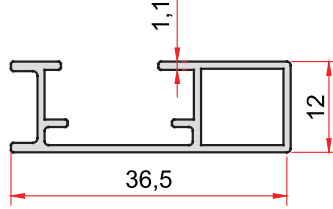
KOD-CODE 1761 TEORİK AĞIRLIK THEORETICAL WEIGHT 0,259 Kg/m
