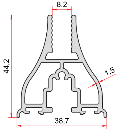
KOD-CODE TEORİK AĞIRLIK THEORETICAL WEIGHT 2291 0,888 Kg/m
