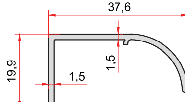
KOD-CODE 1508 TEORİK AĞIRLIK THEORETICAL WEIGHT 0,262 Kg/m
