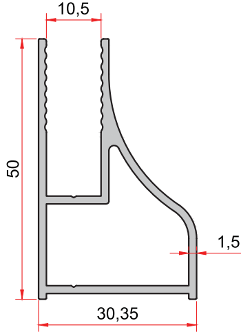
KOD-CODE TEORİK AĞIRLIK 1899 THEORETICAL WEIGHT 0,651 Kg/m
