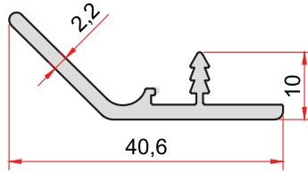
KOD-CODE TEORİK AĞIRLIK THEORETICAL WEIGHT 1474 0,324 Kg/m
