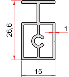
KOD-CODE TEORİK AĞIRLIK 1468 THEORETICAL WEIGHT 0,308 Kg/m
