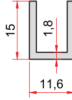
KOD-CODE TEORİK AĞIRLIK 84 THEORETICAL WEIGHT 0,184 Kg/m
