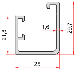
KOD-CODE TEORİK AĞIRLIK 1937 THEORETICAL WEIGHT 0,392 Kg/m
