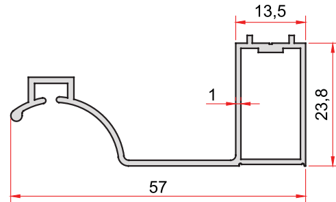
KOD-CODE TEORİK AĞIRLIK THEORETICAL WEIGHT 1781 0,400 Kg/m
