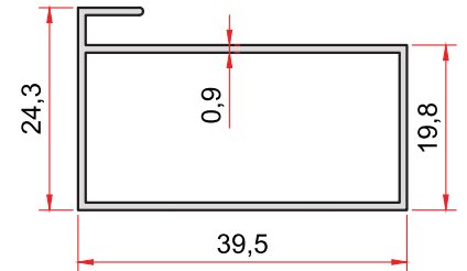
KOD-CODE 1433 TEORİK AĞIRLIK 0,308 Kg/m THEORETICAL WEIGHT
