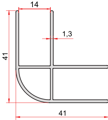
KOD-CODE 1766 TEORİK AĞIRLIK THEORETICAL WEIGHT 0,518 Kg/m
