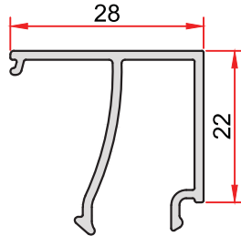
KOD-CODE TEORİK AĞIRLIK CC-1180-13 THEORETICAL WEIGHT 0,300 Kg/m
