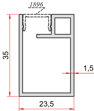
KOD-CODE 5052 TEORİK AĞIRLIK 0,488 Kg/m THEORETICAL WEIGHT
