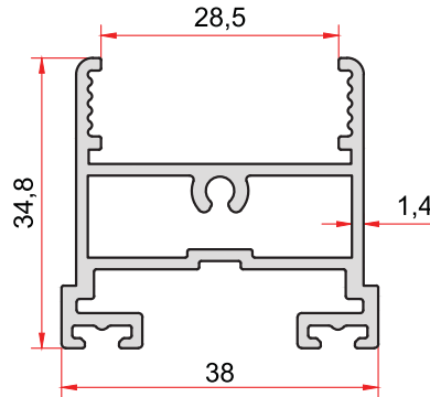
KOD-CODE 2634 TEORİK AĞIRLIK THEORETICAL WEIGHT 0,726 Kg/m
