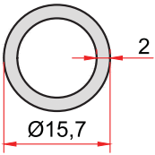
KOD-CODE 1893 TEORİK AĞIRLIK THEORETICAL WEIGHT 0,232 Kg/m
