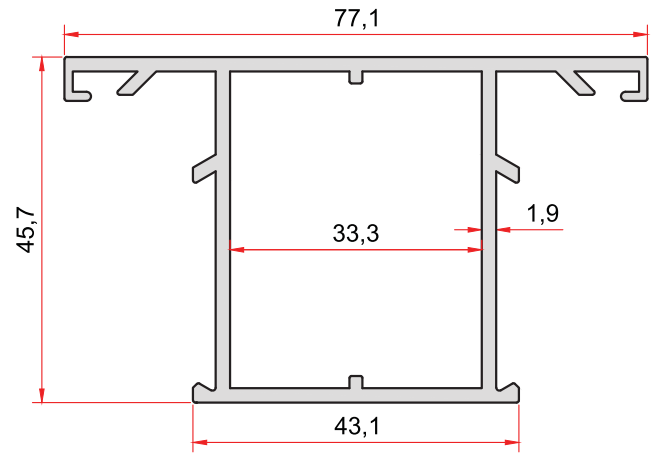
KOD-CODE TEORİK AĞIRLIK 880 THEORETICAL WEIGHT 1,177 Kg/m
