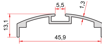
KOD-CODE 863 TEORİK AĞIRLIK THEORETICAL WEIGHT 0,310 Kg/m
