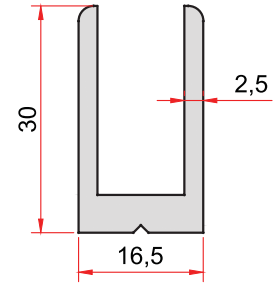
KOD-CODE 841 TEORİK AĞIRLIK THEORETICAL WEIGHT 0,553 Kg/m
