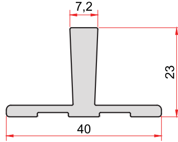
KOD-CODE 1473 TEORİK AĞIRLIK THEORETICAL WEIGHT 0,618 Kg/m
