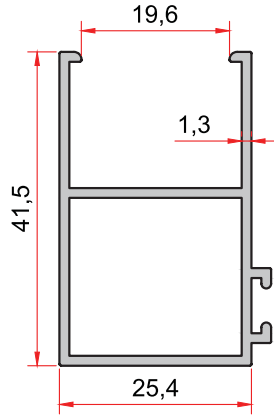
KOD-CODE 1088 TEORİK AĞIRLIK THEORETICAL WEIGHT 0,489 Kg/m
