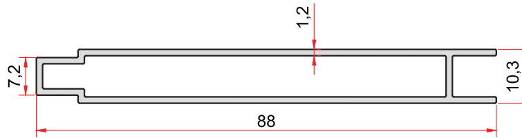
KOD-CODE TEORİK AĞIRLIK 1035 THEORETICAL WEIGHT 0,622 Kg/m
