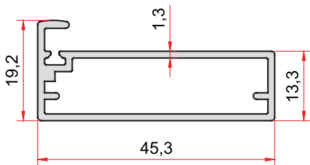
KOD-CODE 1384 TEORİK AĞIRLIK 0,475 Kg/m THEORETICAL WEIGHT
