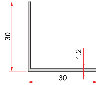
KOD-CODE 16 TEORİK AĞIRLIK THEORETICAL WEIGHT 0,192 Kg/m
