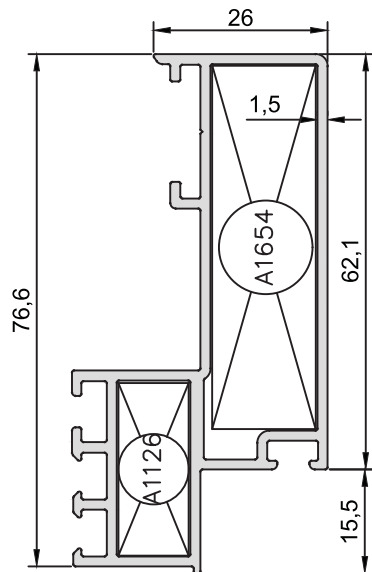
KOD-CODE AF-5065-15 TEORİK AĞIRLIK THEORETICAL WEIGHT 1,135 Kg/m
