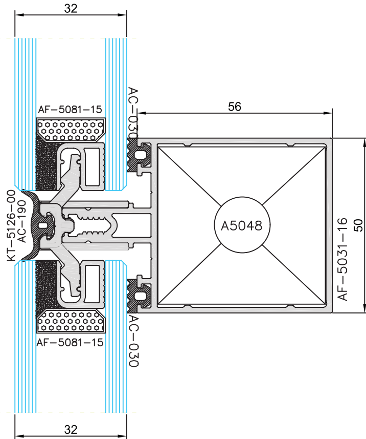
Silikon Cephe Cam Klipsi Detayı
