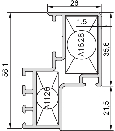
KOD-CODE AF-5067-15 TEORİK AĞIRLIK THEORETICAL WEIGHT 0,880 Kg/m
