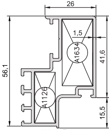
*Mat Eloksal KOD-CODE AF-5061-15 TEORİK AĞIRLIK THEORETICAL WEIGHT 0,880 Kg/m
