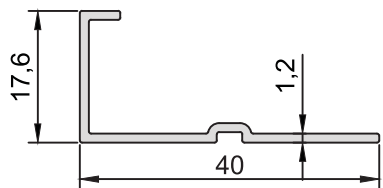
KOD-CODE TEORİK AĞIRLIK AF-5097-12 THEORETICAL WEIGHT 0,206 Kg/m
