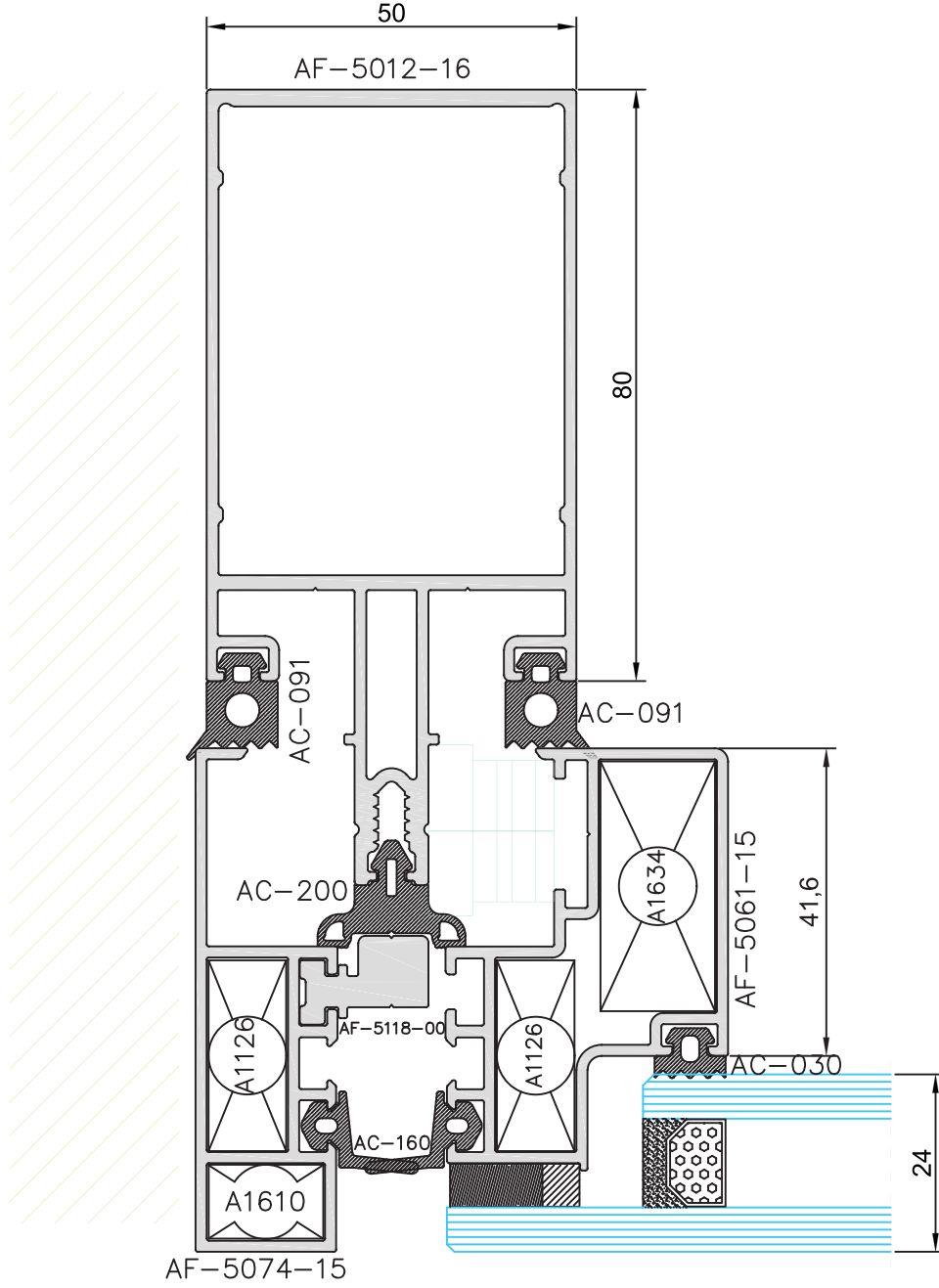
Silikon Cephe Bitiş Detayı
