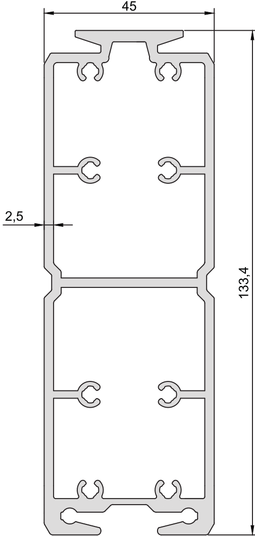
KOD-CODE TEORİK AĞIRLIK KT-5133-00 THEORETICAL WEIGHT 3,467 Kg/m
