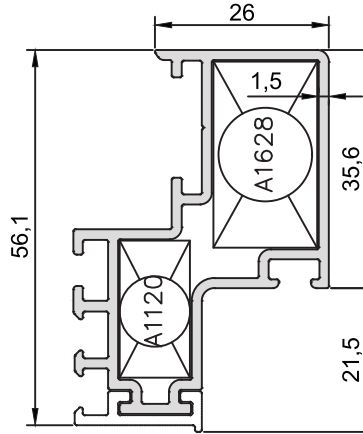
KOD-CODE AF-5068-15 TEORİK AĞIRLIK THEORETICAL WEIGHT 0,852 Kg/m
