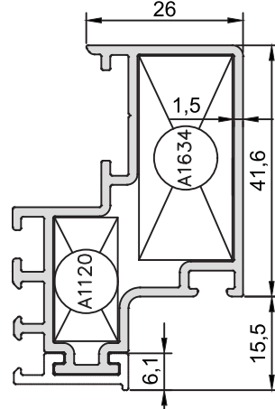
KOD-CODE AF-5062-15 TEORİK AĞIRLIK THEORETICAL WEIGHT 0,852 Kg/m
